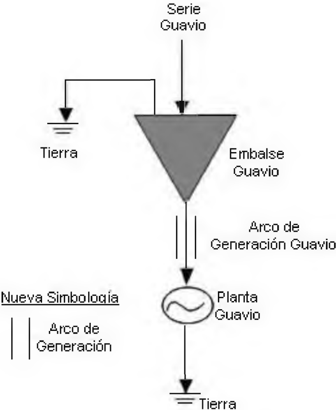
Diagrama Topológico Guavio
