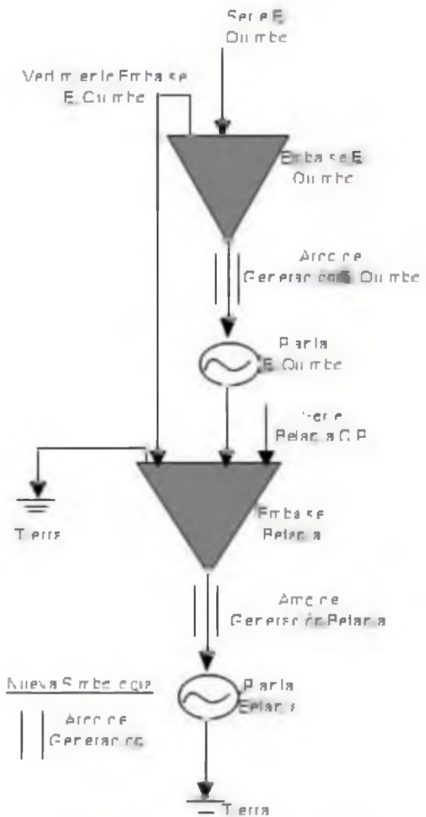
Diagrama Topológico Quimbo – Betania
