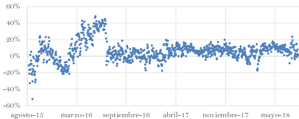
Figura 15. Desviaciones de plantas menores entre la generación programada y la generación real; datos de XM
