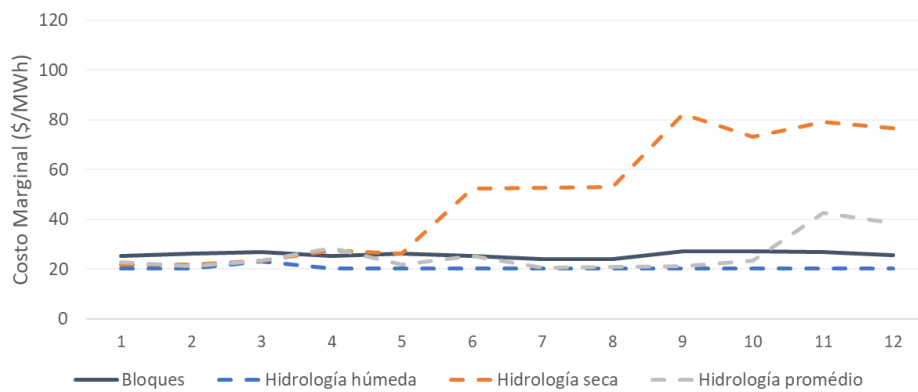
Figura 133 – Escenario con elevada GD, Costos marginales horarios (2025).
