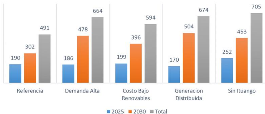
Figura 163 – Líneas Construidas [Km] para cada año y escenario.
