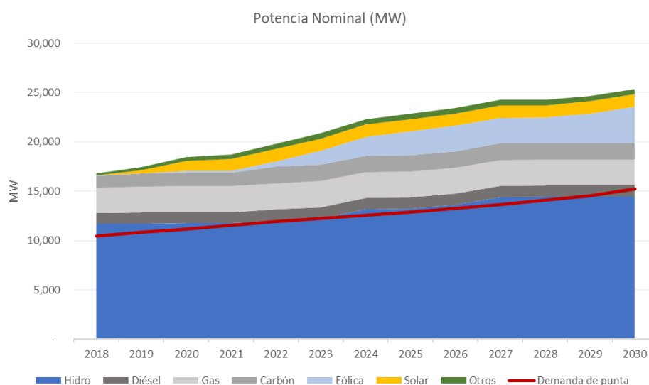
Figura 59 – Balance de Potencia por año – Escenario de Referencia.
