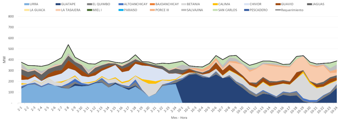
Figura 76 – Asignación de la reserva operativa (2025).
