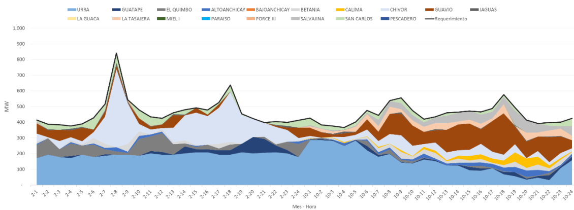
Figura 77 – Asignación de la reserva operativa (2030).
