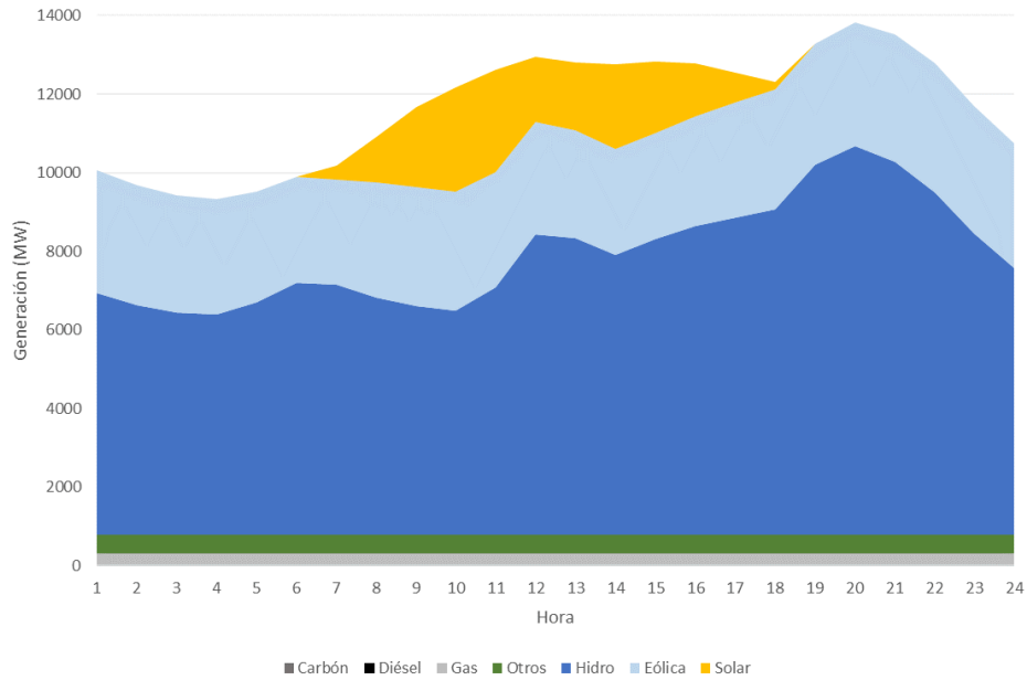
Figura 111 – Escenario sin Pescadero, Balance Diario (Junio 2030, Hidrología Promedio).
