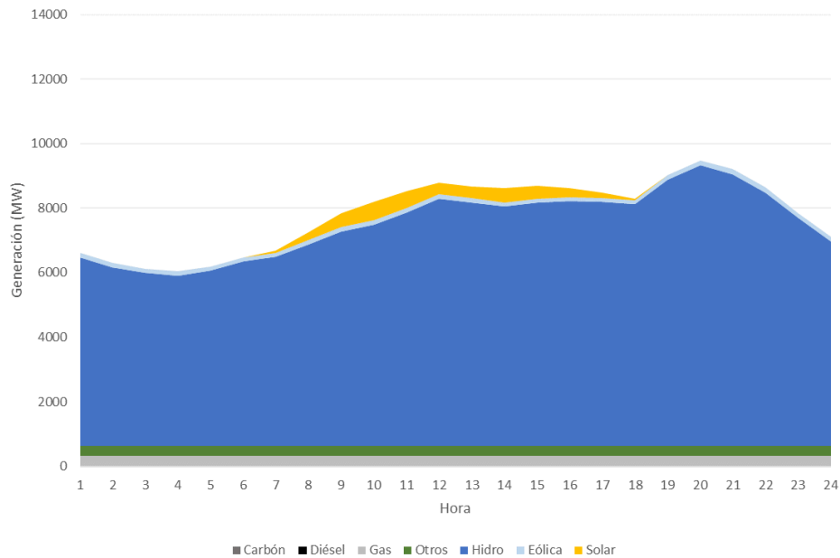
Figura 107 – Escenario sin Pescadero, Balance Diario (Junio 2021, Hidrología Promedio).
