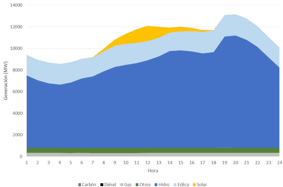
Figura 93 – Demanda Alta – Diciembre 2030, Hidrología Promedio
