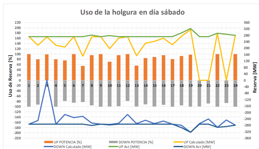
Figura 166 – Holgura AGC en días sábado
