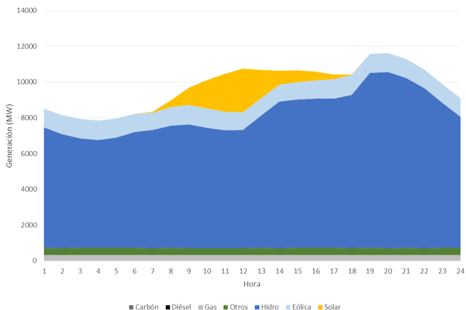
Figura 148 – Escenario precios bajos renovables, Balance Diario (Diciembre 2025, Hidrología Promedio).
