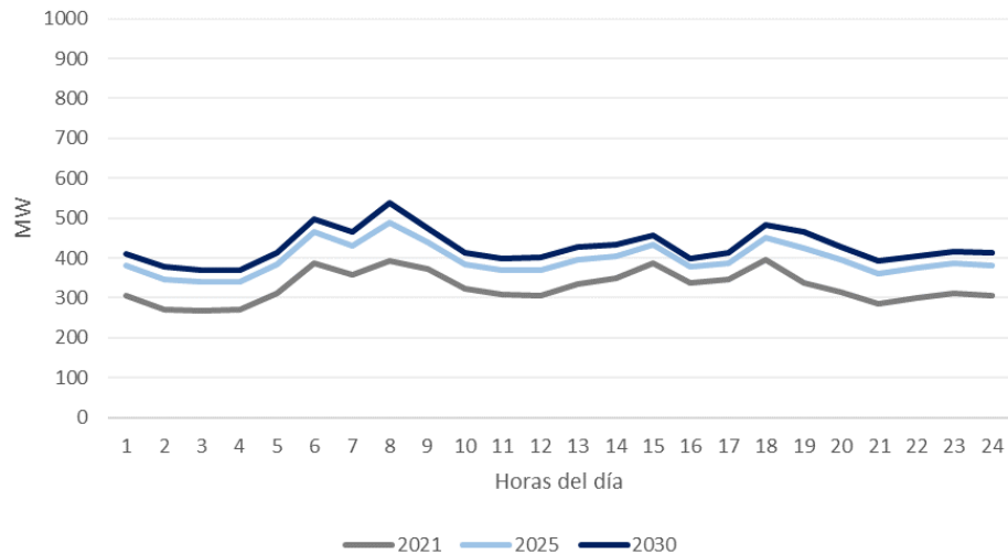
Figura 62 – Requerimientos de reserva en giro para la imprevisibilidad de las ERVs.
