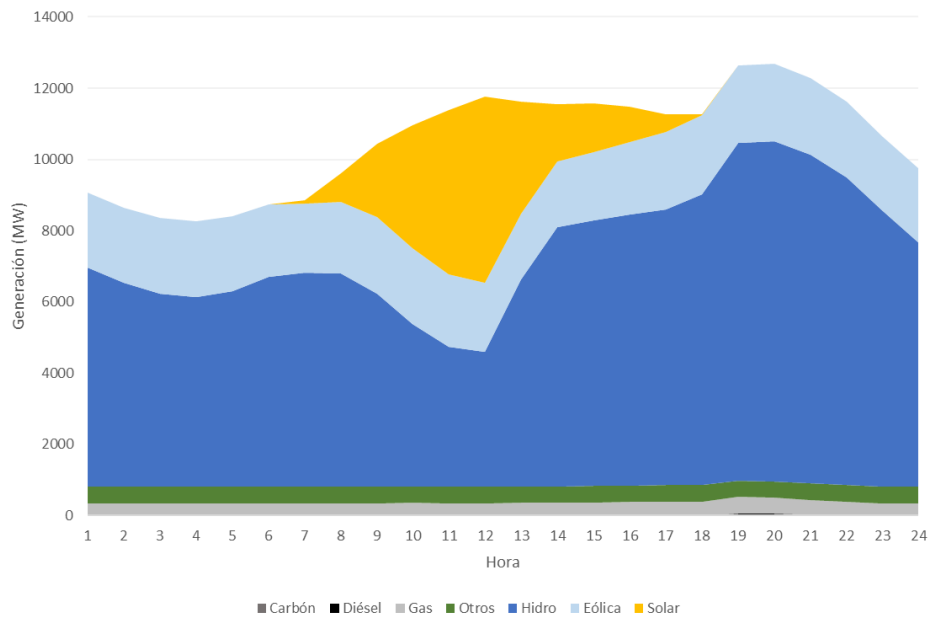
Figura 112 – Escenario sin Pescadero, Balance Diario (Diciembre 2030, Hidrología Promedio).
