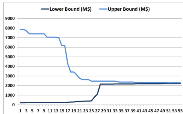
Figura 191 – Expansión integrada G&T Bolivia – convergencia de la descomposición de Benders
