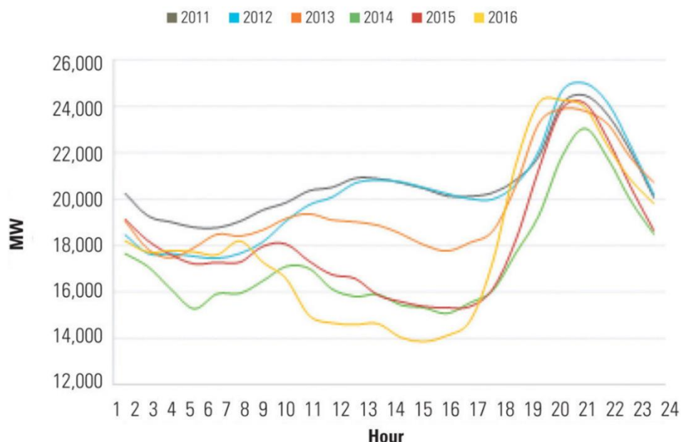
Figura 29 – Demanda neta (California): demanda electricidad – producción renovable
