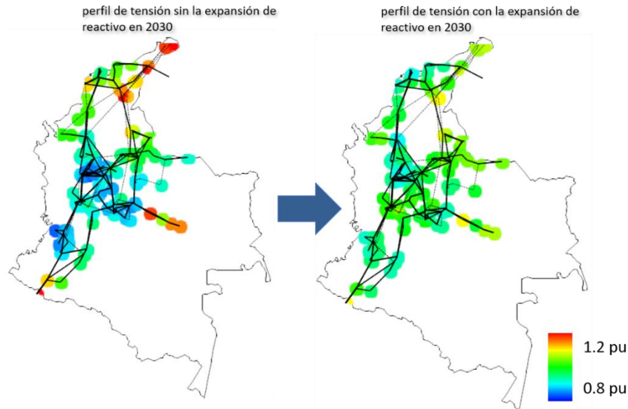
Figura 66 – Perfil de tensión sin la expansión x con la expansión en 2030 para el escenario de referencia (Escenario Promedio, Diciembre).
