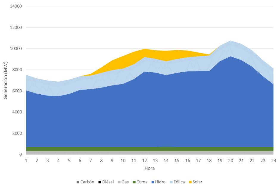
Figura 109 – Escenario sin Pescadero, Balance Diario (Junio 2025, Hidrología Promedio).
