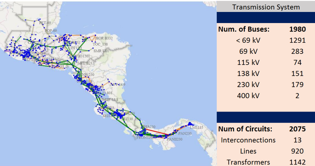
Figura 194 – sistema de transmisión de Centro América
