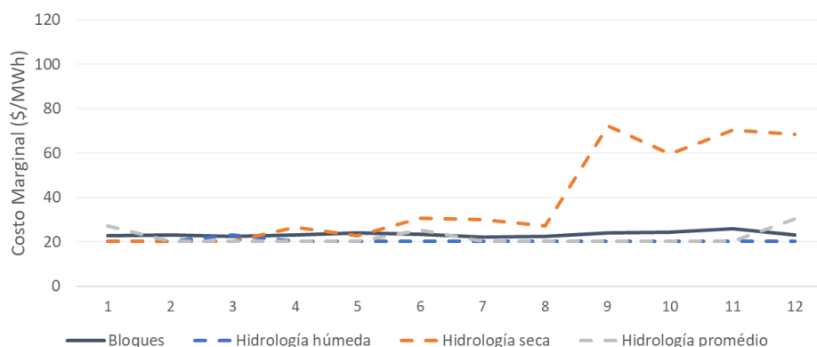
Figura 152 – escenario precios bajos renovables, Costos marginales horarios (2025).
