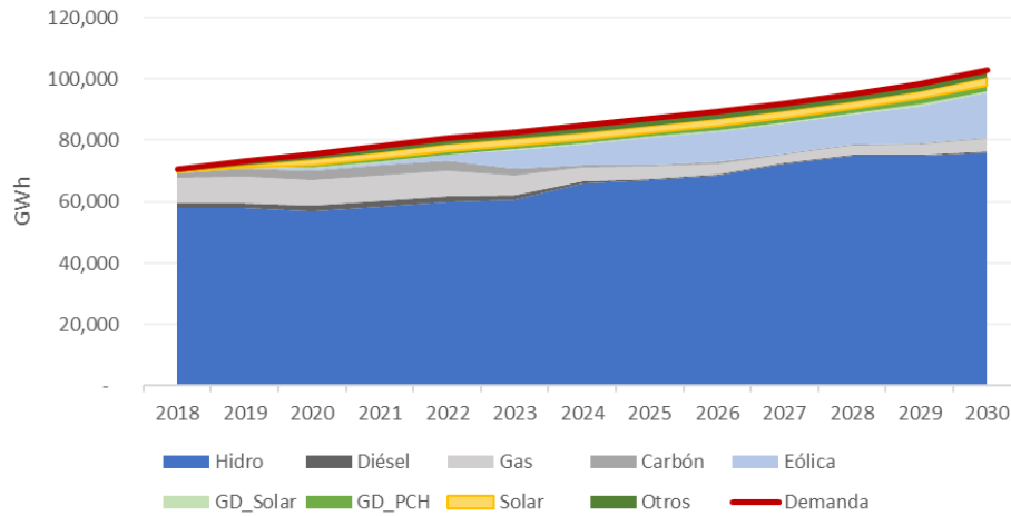
Figura 120 – Balance de Generación – Escenario con elevada GD
