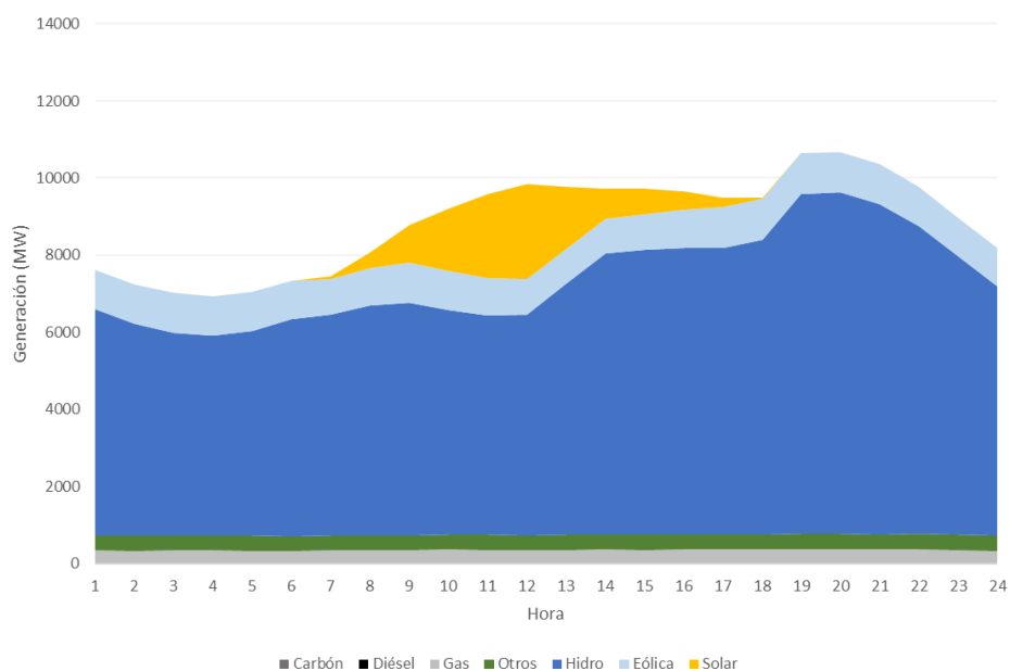
Figura 110 – Escenario sin Pescadero, Balance Diario (Diciembre 2025, Hidrología Promedio).
