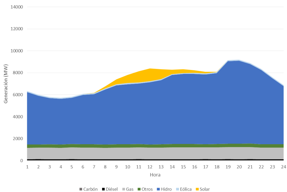
Figura 89 – Demanda Alta – Diciembre 2021, Hidrología Promedio
