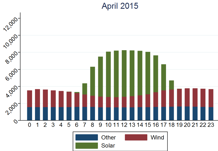
Figura 27 – Perfil diario típico de producción (California) - 2015
