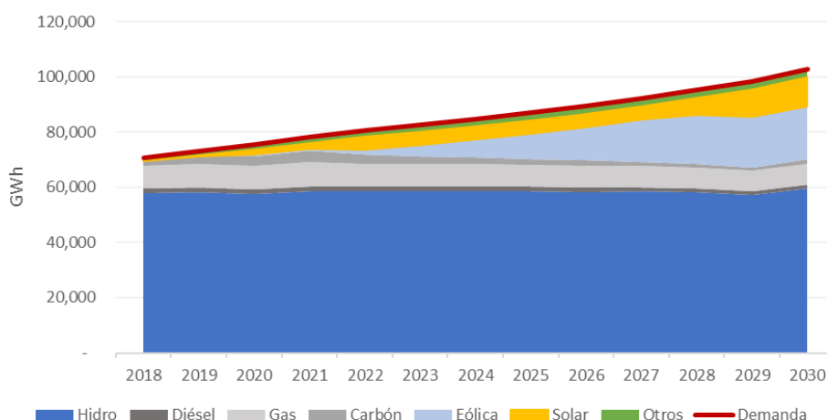
Figura 101 – Balance de Generación – Escenario sin Pescadero.
