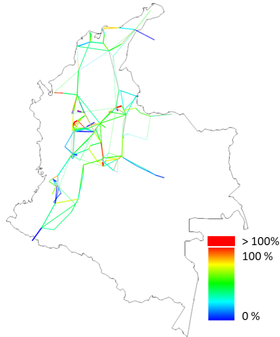
Figura 63 – flujo máximo en 2030 para el escenario de referencia.
