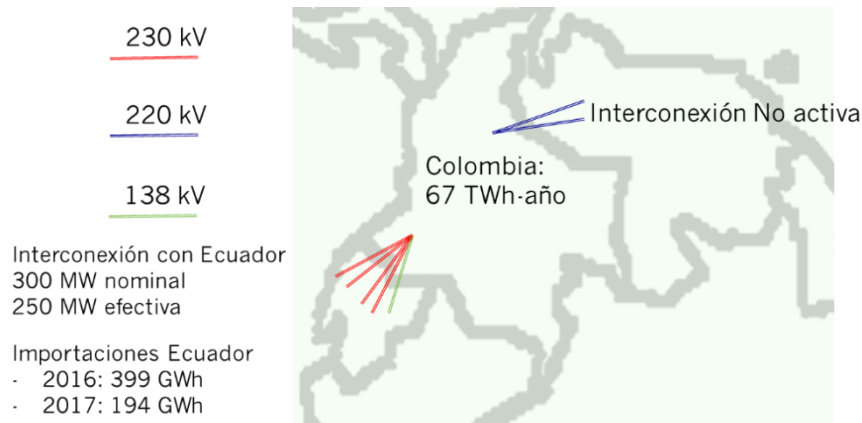
Figura 6 – Líneas de transmisión – interconexiones internacionales
