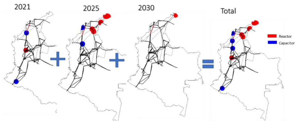
Figura 65 – Resultado de la expansión de reactivo para el escenario de referencia.
