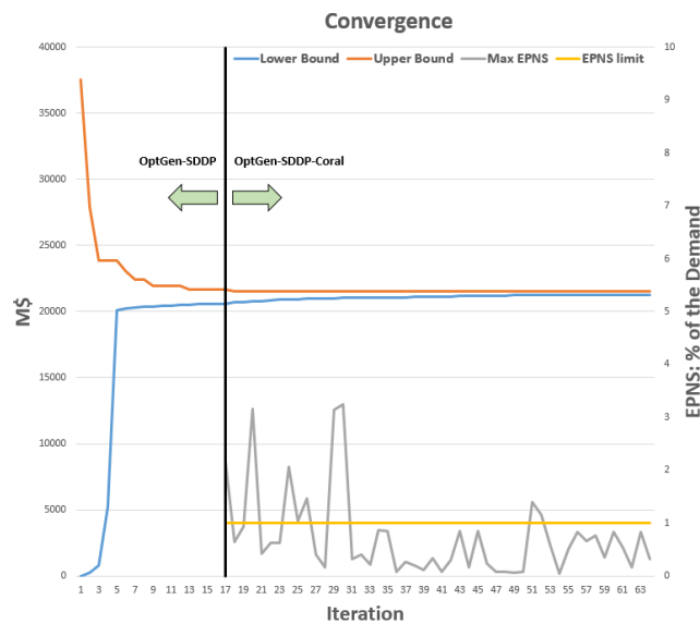
Figura 193 – Expansión Marruecos – convergencia de la descomposición de Benders
