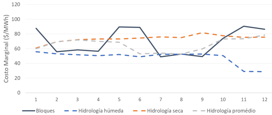
Figura 94 – Costos marginales horarios, 2021
