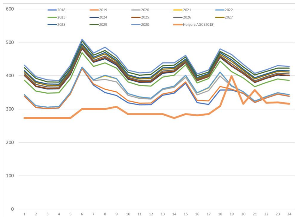
Figura 171 – Reserva operativa calculada por la suma de las 3 componentes
