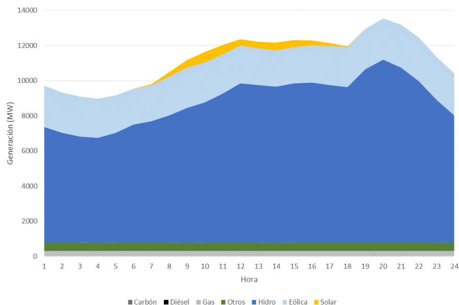
Figura 130 – Escenario con elevada GD, Balance Diario (Junio 2030, Hidrología Promedio).
