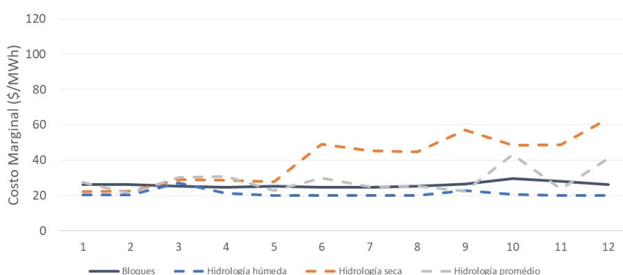
Figura 75 – Escenario de Referencia, Costos marginales horarios (2030).
