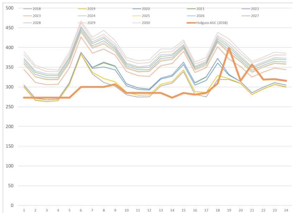
Figura 173 – Reserva operativa ajustando las 3 componentes para la holgura propuesta por XM para el año 2018
