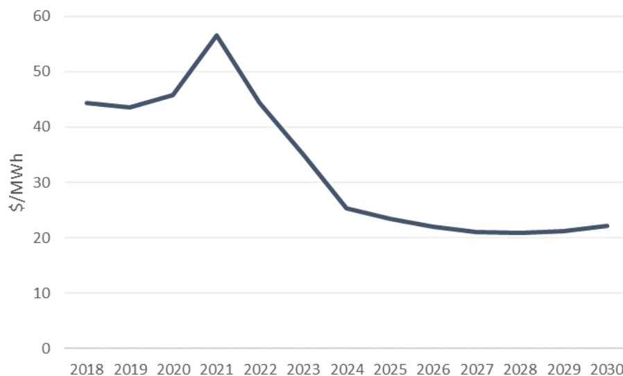
Figura 138 - Costos Marginales Anuales – escenario precios bajos renovables.
