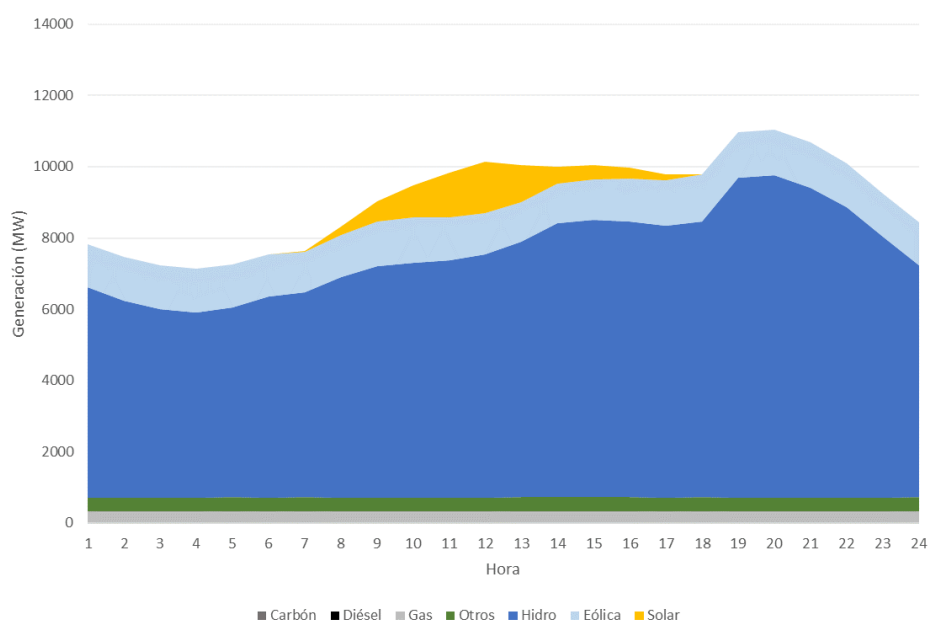
Figura 91 – Demanda Alta – Diciembre 2025, Hidrología Promedia
