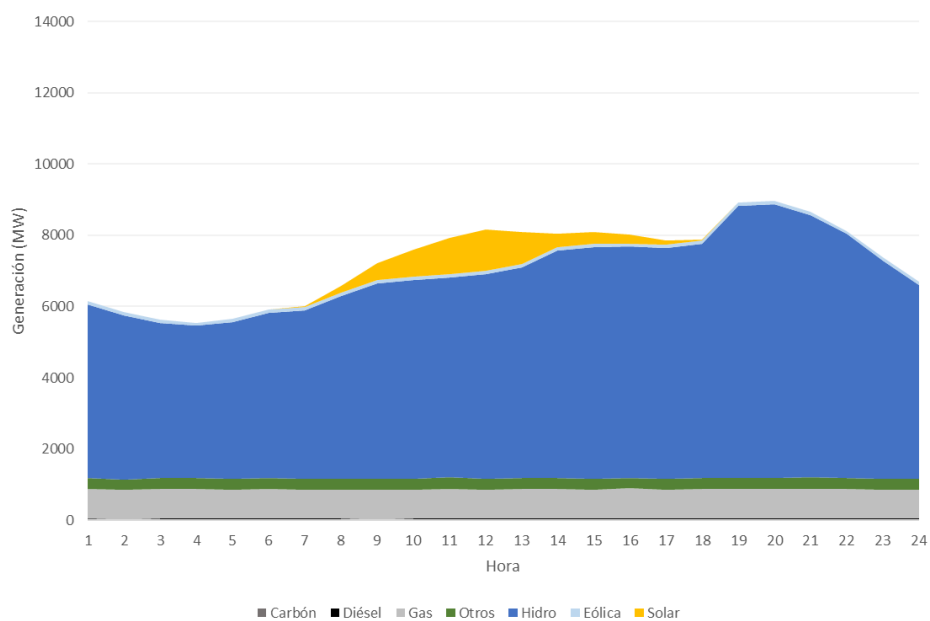
Figura 68 – Escenario de Referencia, Balance Diario (Diciembre 2021, Hidrología Promedio).
