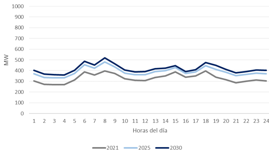
Figura 121 – Requerimientos de reserva en giro para la imprevisibilidad de las ERVs.
