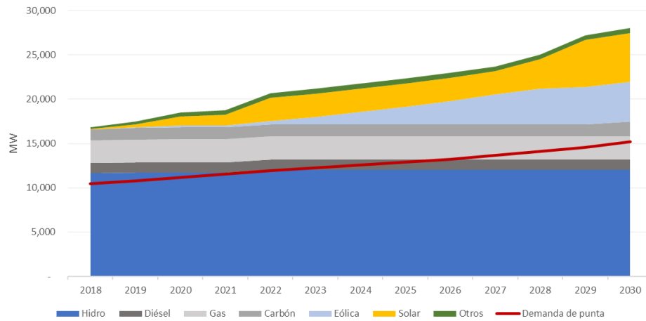
Figura 99 – Balance de Potencia por año – Escenario sin Pescadero.
