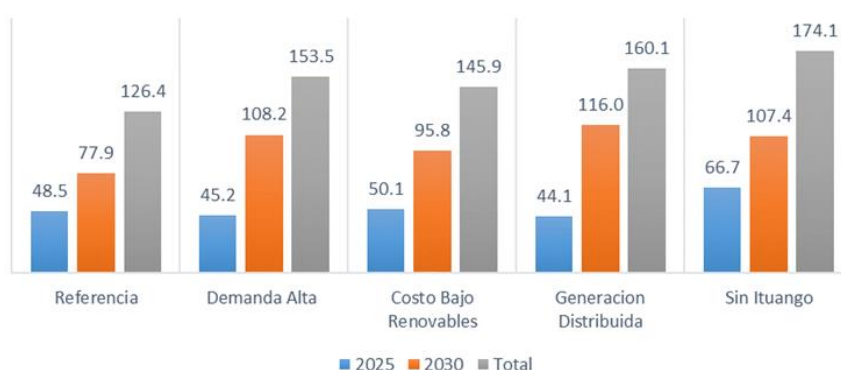
Figura 164 – Costo de Inversión [M$] para transmisión para cada año y escenario.
