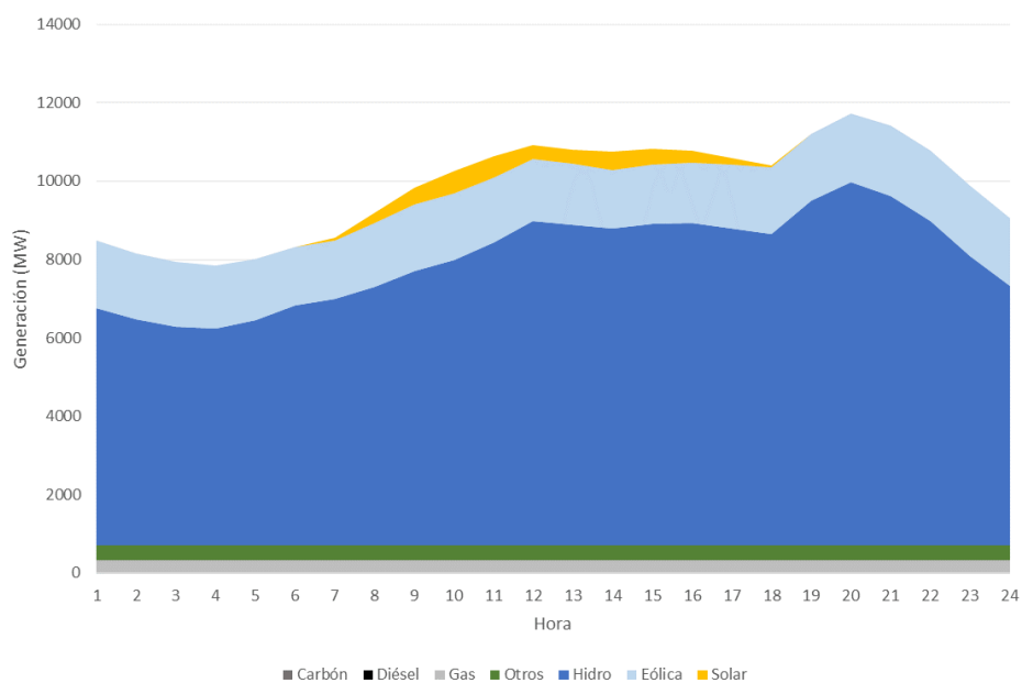
Figura 69 – Escenario de Referencia, Balance Diario (Junio 2025, Hidrología Promedio).
