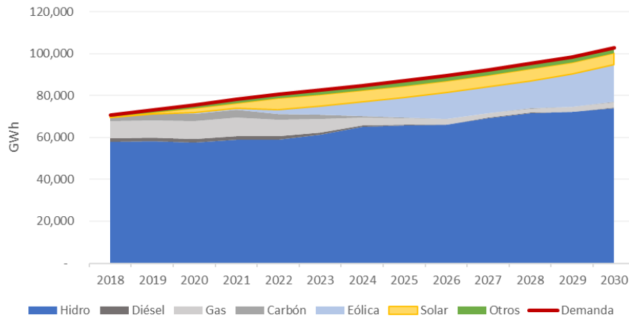
Figura 139 – Balance de Generación – escenario precios bajos renovables.
