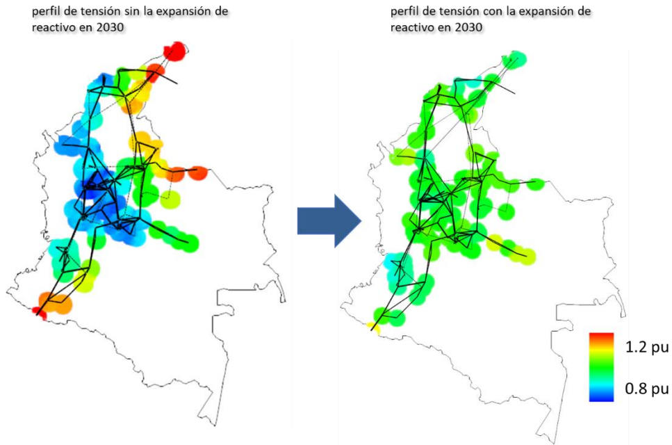
Figura 144 – Perfil de tensión sin la expansión x con la expansión en 2030 para el escenario de inserción agresiva de costo bajo de inversión para las renovables (Escenario Promedio, Diciembre).
