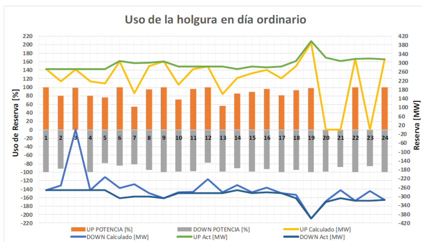
Figura 16 – Holgura AGC en días ordinarios
