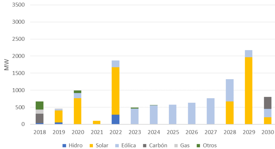
Figura 97 – Adición de capacidad por año – Escenario sin Pescadero.
