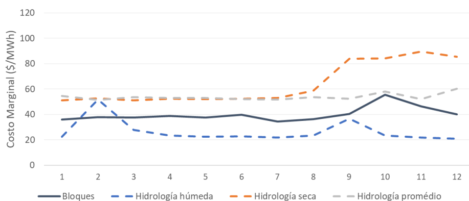
Figura 114 – Escenario sin Pescadero, Costos marginales horarios (2025).
