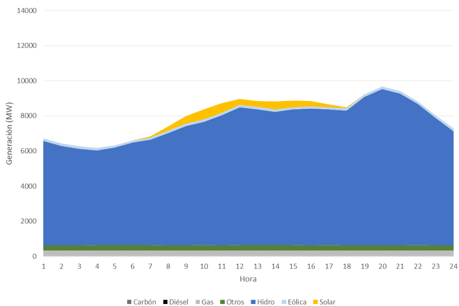
Figura 88 – Demanda Alta – Junio 2021, Hidrología Promedio
