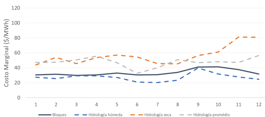
Figura 115 – Escenario sin Pescadero, Costos marginales horarios (2030).
