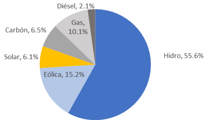
Figura 79 - Cap. Inst. – Escenario demanda alta (2030).
