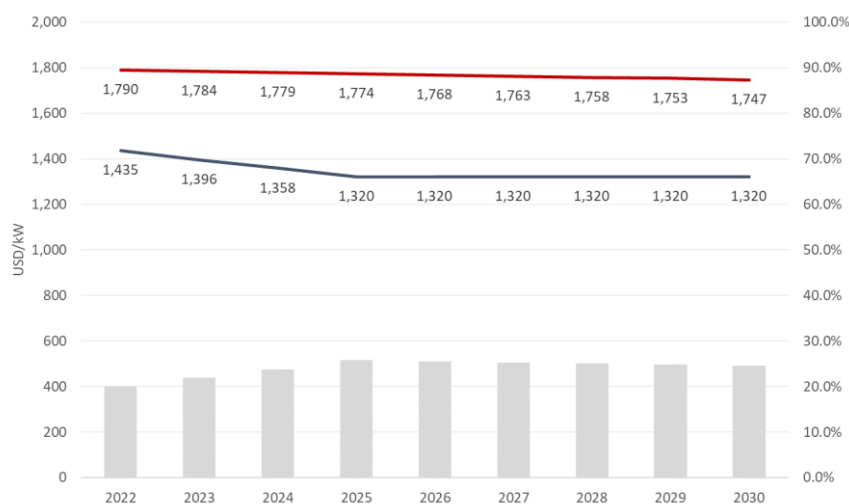
Figura 50 – Costos de inversión de las centrales eólicas 9 .
