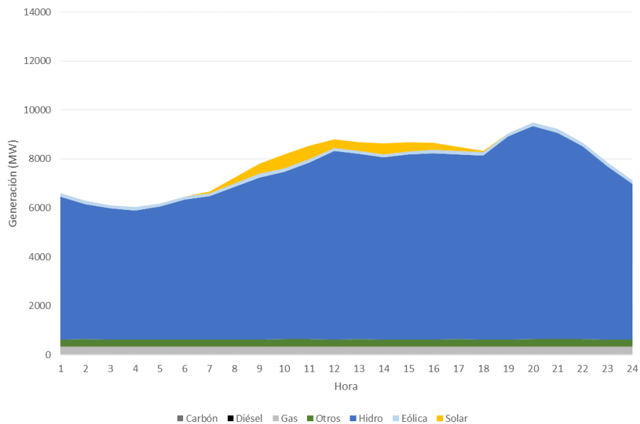
Figura 145 – Escenario precios bajos renovables, Balance Diario (Junio 2021, Hidrología Promedio).
