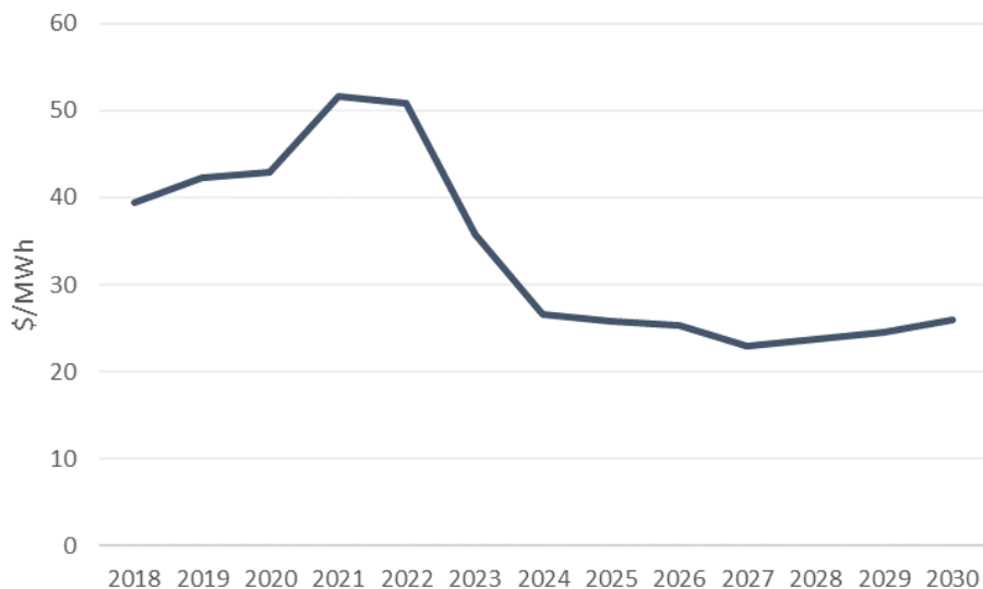
Figura 119 - Costos Marginales Anuales – Escenario con elevada GD
