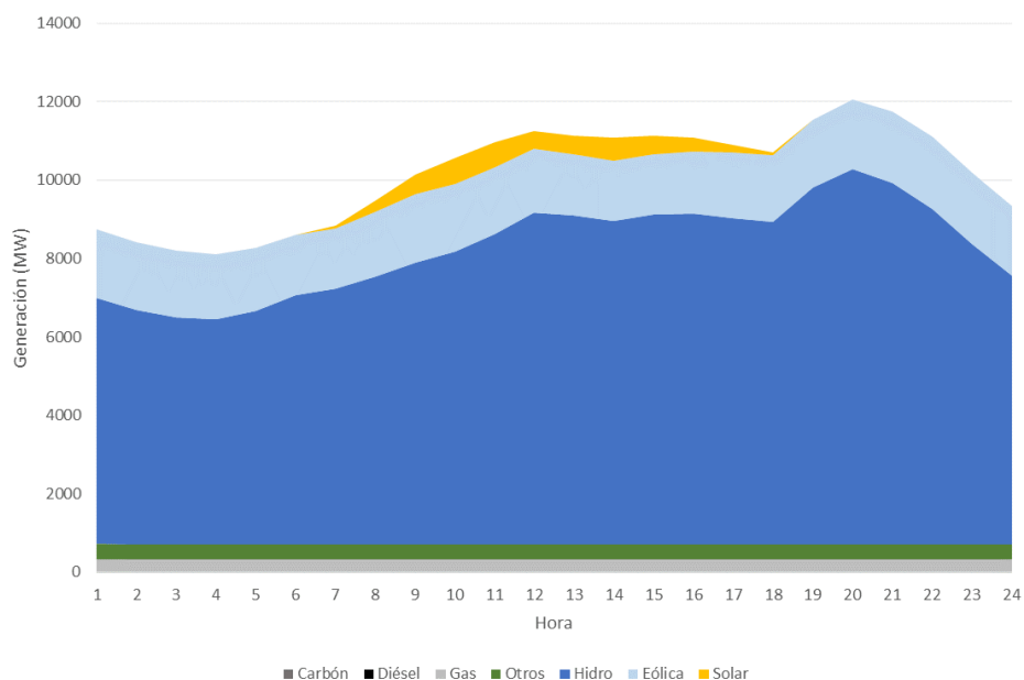
Figura 90 – Demanda Alta – Junio 2025, Hidrología Promedio
