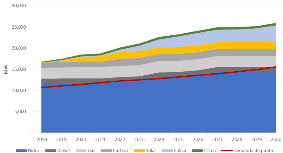
Figura 80 – Balance de Potencia por año – Escenario demanda alta.
