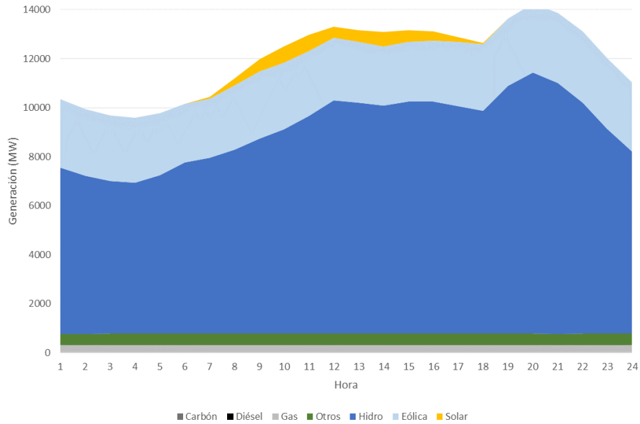
Figura 92 – Demanda Alta – Junio 2030, Hidrología Promedio
