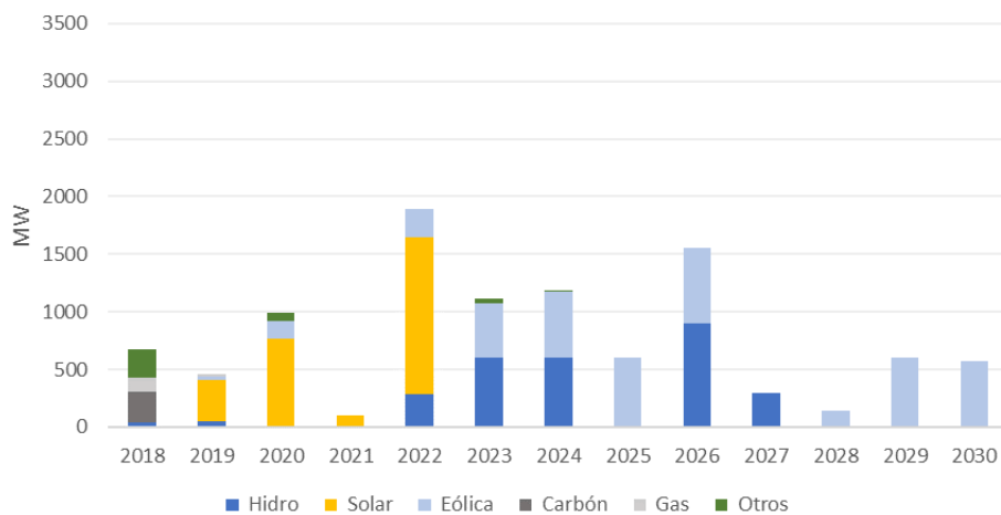
Figura 135 – Adición de capacidad por año – escenario Costo Bajo renovables.
