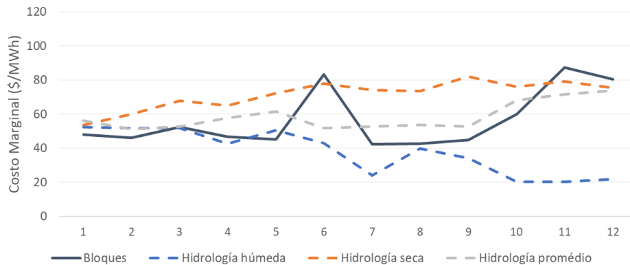
Figura 151 – escenario precios bajos renovables, Costos marginales horarios (2021).
