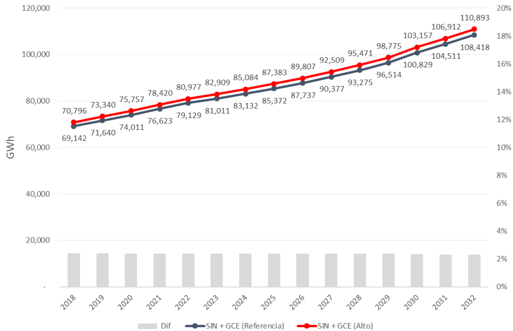
Figura 44 - Proyección de Demanda - Colombia.
