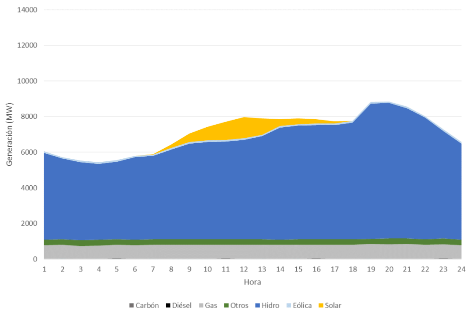
Figura 127 – Escenario con elevada GD, Balance Diario (Diciembre 2021, Hidrología Promedio).
