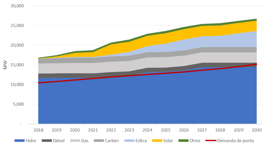
Figura 137 – Balance de Potencia por año – escenario precios bajos renovables.
