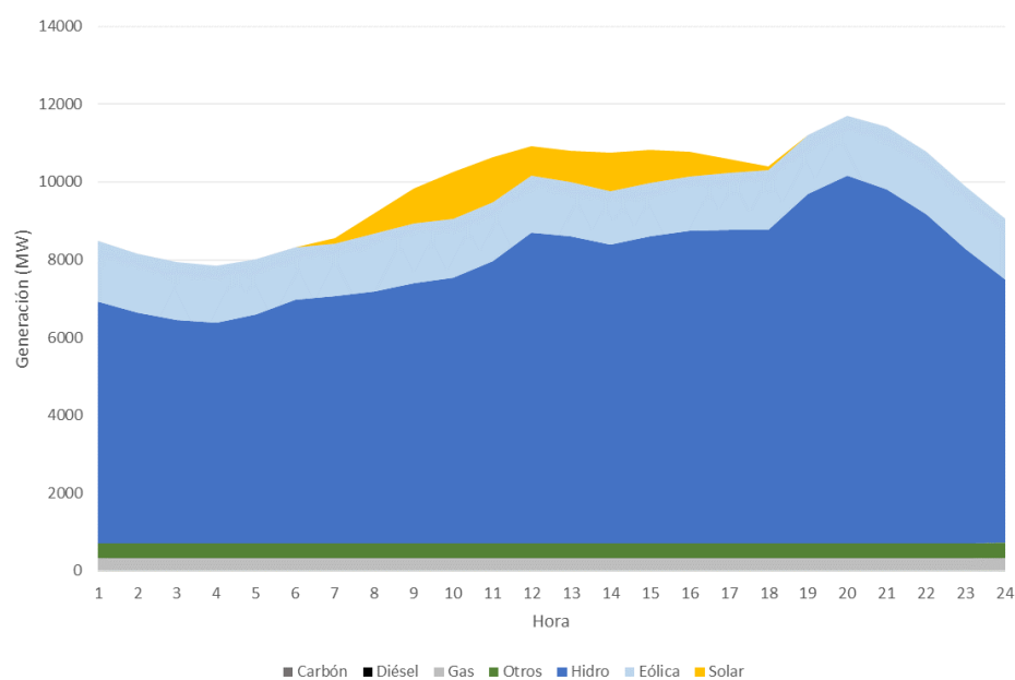
Figura 147 – Escenario precios bajos renovables, Balance Diario (Junio 2025, Hidrología Promedio).
