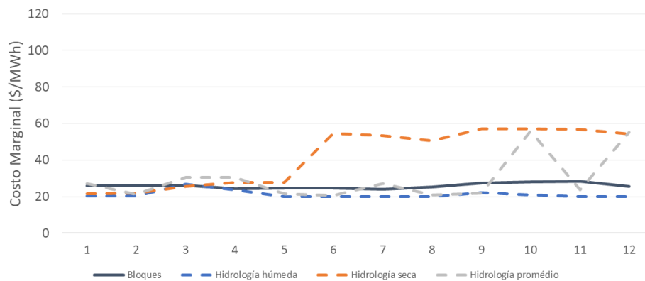
Figura 134 – Escenario con elevada GD, Costos marginales horarios (2030).
