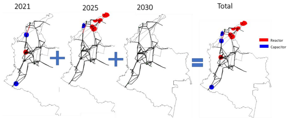
Figura 86 – Resultado de la expansión de reactivo para el escenario de demanda alta.
