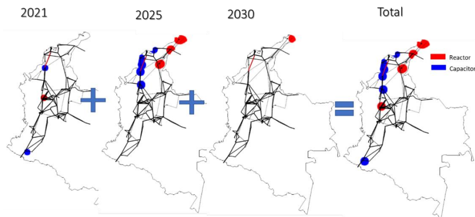
Figura 105 – Resultado de la expansión de reactivo para el escenario sin Pescadero/Ituango.
