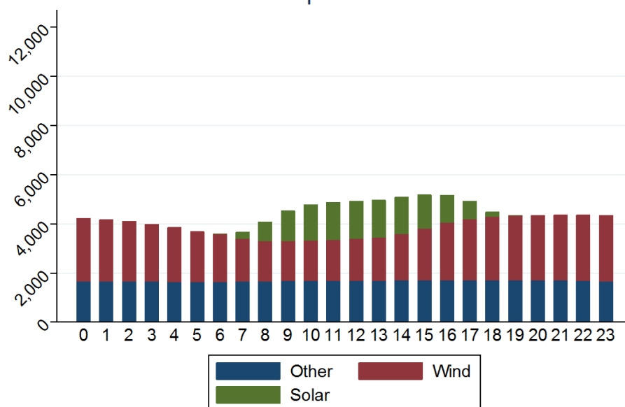
Figura 26 – Perfil diario típico de producción (California) - 2013
