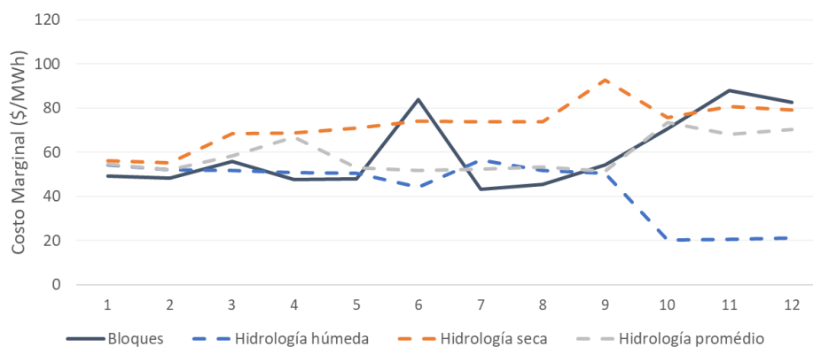
Figura 113 – Escenario sin Pescadero, Costos marginales horarios (2021).
