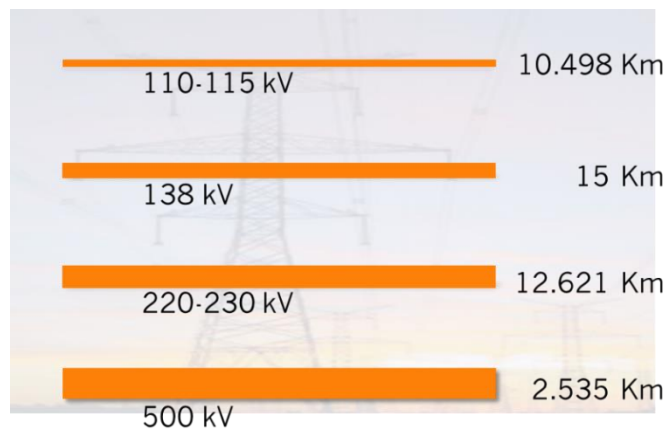
Figura 5 – Longitud de las líneas de transmisión (por voltaje)
