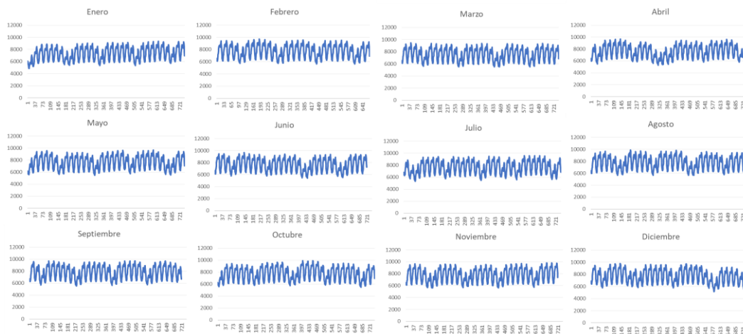
Figura 45 – Perfil de demanda horaria para el sistema de Colombia.
