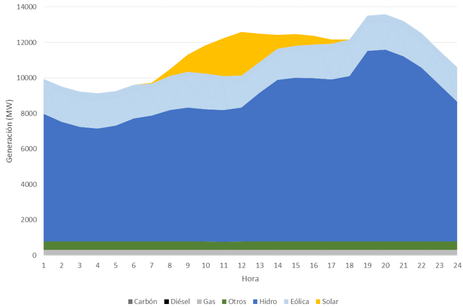
Figura 150 – Escenario precios bajos renovables, Balance Diario (Diciembre 2030, Hidrología Promedio).
