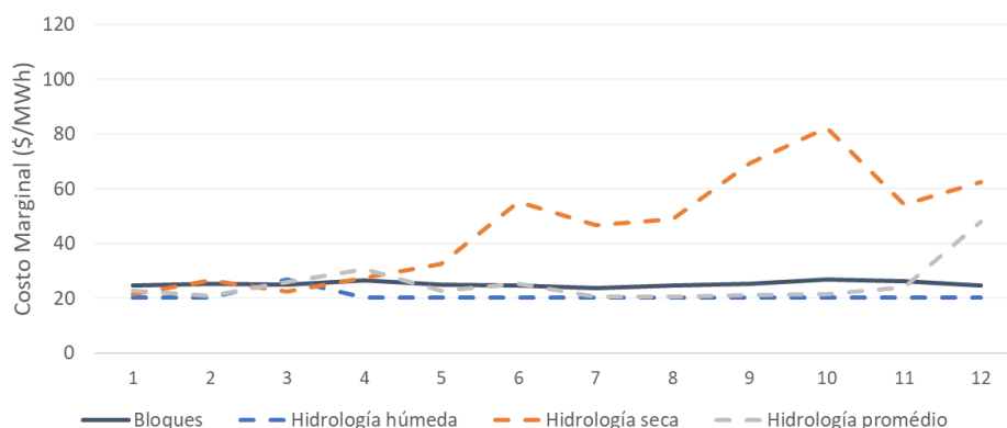
Figura 74 – Escenario de Referencia, Costos marginales horarios (2025).
