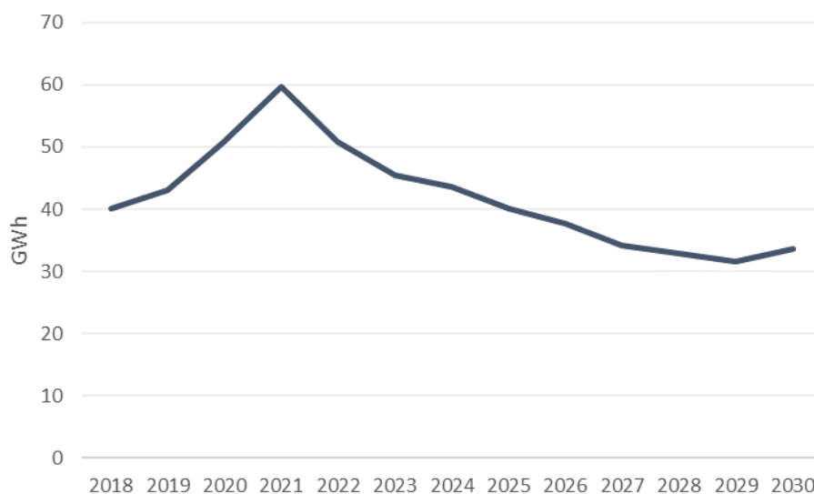
Figura 100 - Costos Marginales Anuales – Escenario sin Pescadero.
