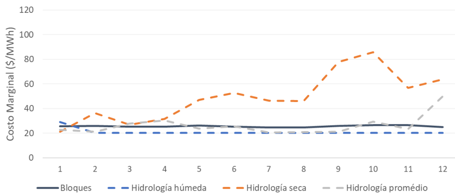
Figura 95 – Costos marginales horarios, 2025
