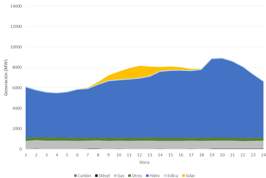
Figura 146 – Escenario precios bajos renovables, Balance Diario (Diciembre 2021, Hidrología Promedio).
