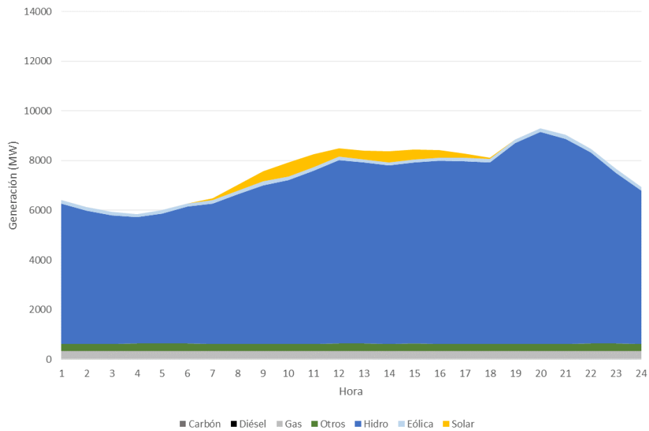
Figura 126 – Escenario con elevada GD, Balance Diario (Junio 2021, Hidrología Promedio).
