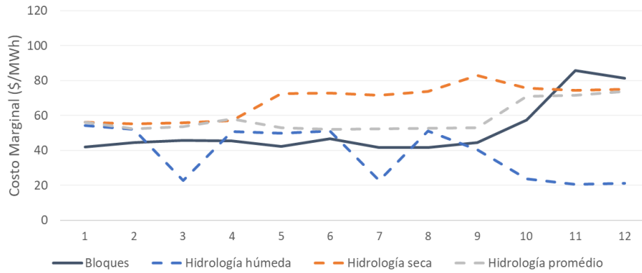
Figura 132 – Escenario con elevada GD, Costos marginales horarios (2021).
