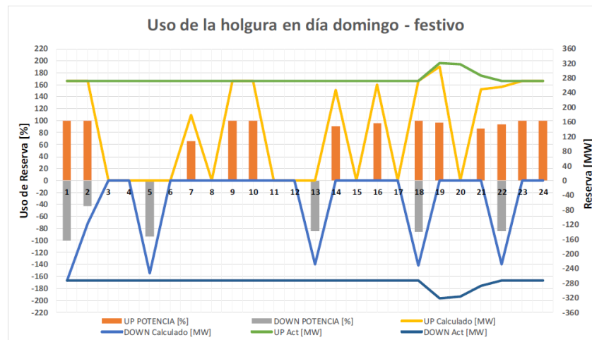
Figura 18 – Holgura en Domingos y Festivos
