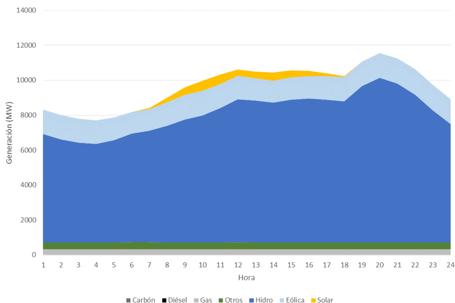
Figura 128 – Escenario con elevada GD, Balance Diario (Junio 2025, Hidrología Promedio).
