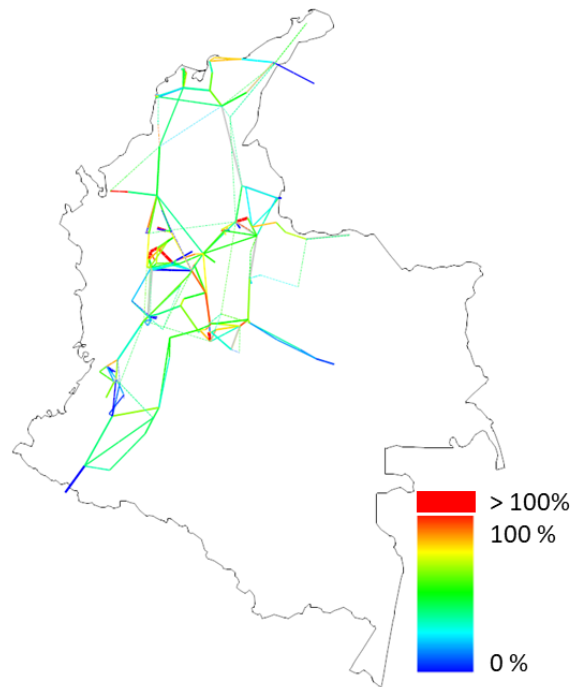
Figura 84 – flujo máximo en 2030 para el escenario de demanda alta.
