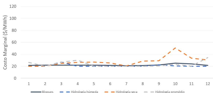
Figura 153 – escenario precios bajos renovables, Costos marginales horarios (2030).
