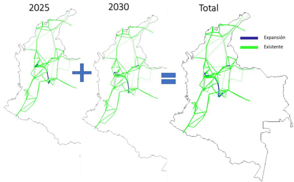
Figura 85 – Resultado de la expansión de transmisión para el escenario de demanda alta.
