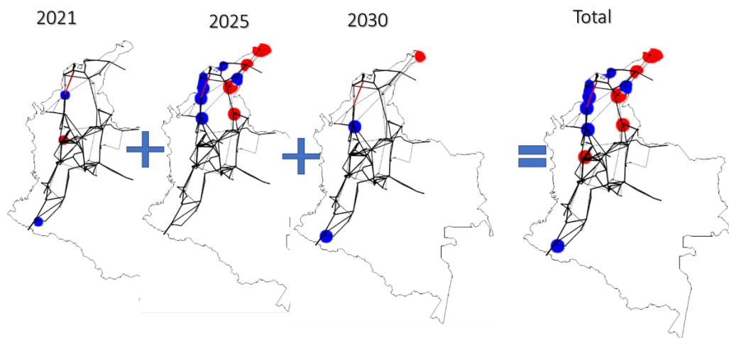
Figura 143 – Resultado de la expansión de reactivo para el escenario inserción agresiva de costo bajo de inversión para las renovables.
