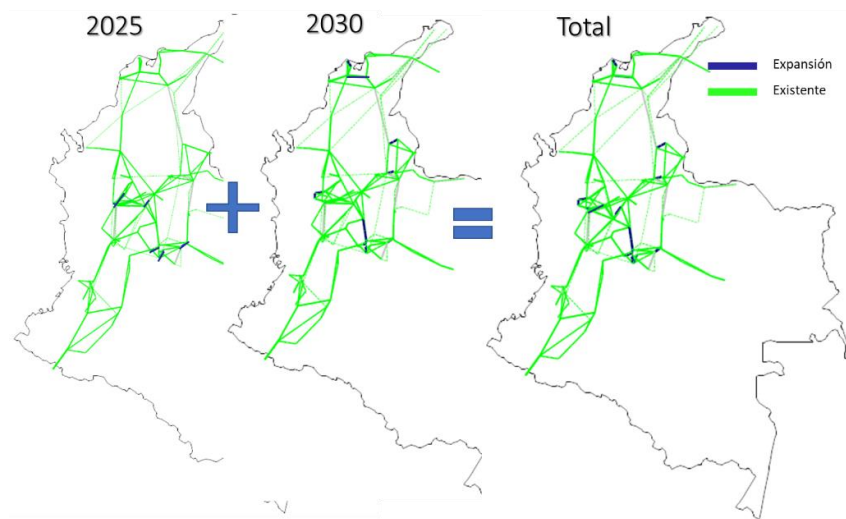
Figura 104 – Resultado de la expansión de transmisión para el escenario sin Pescadero/Ituango.
