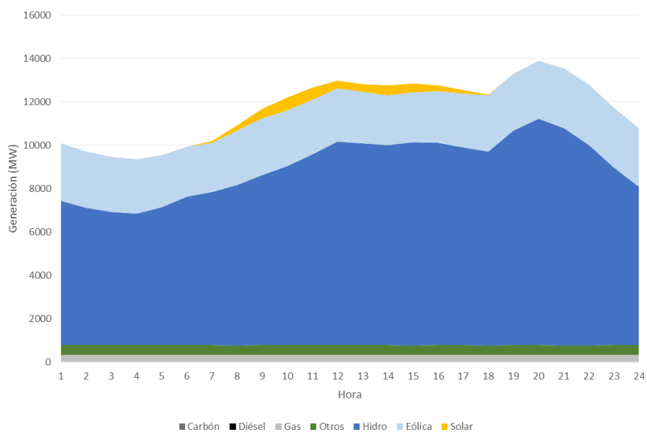
Figura 71 – Escenario de Referencia, Balance Diario (Junio 2030, Hidrología Promedio).
