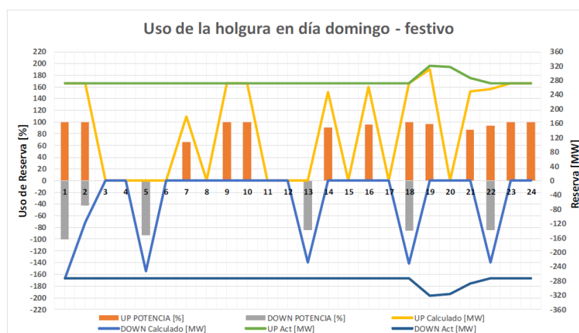
Figura 167 – Holgura en Domingos y Festivos
