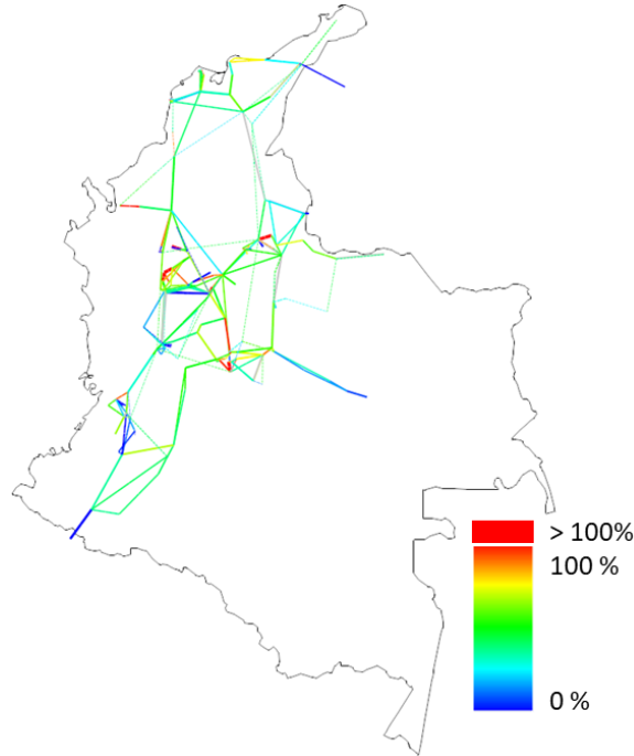
Figura 122 – flujo máximo en 2030 para el escenario de inserción agresiva de generación distribuida.
