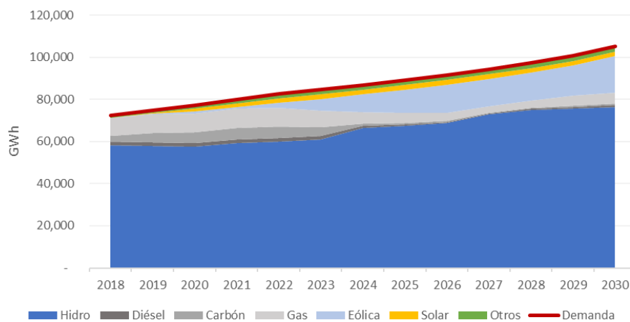
Figura 82 – Balance de Generación – Escenario demanda alta.
