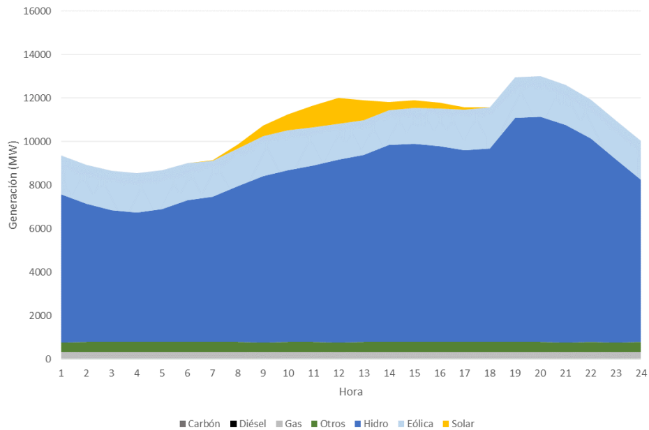
Figura 72 – Escenario de Referencia, Balance Diario (Diciembre 2030, Hidrología Promedio).
