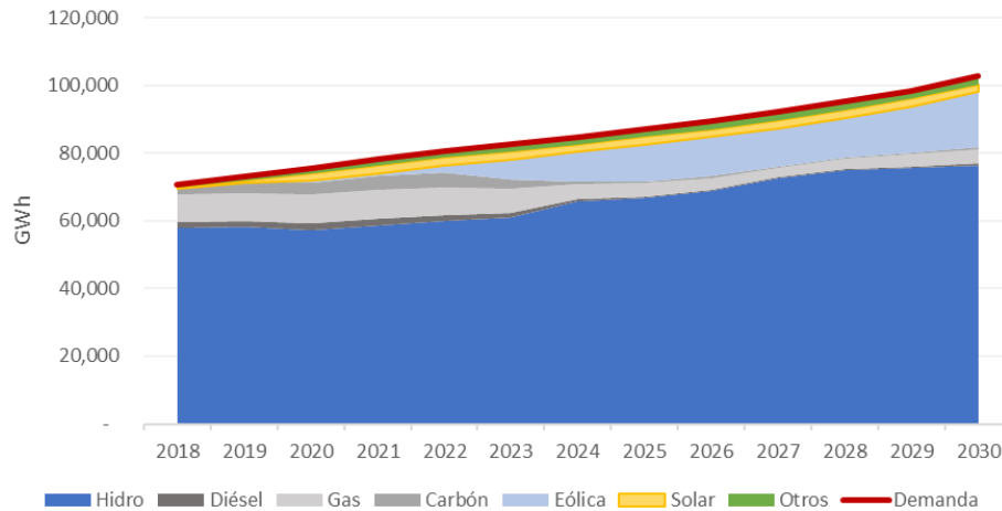
Figura 61 – Balance demanda x generación – Escenario de Referencia.
