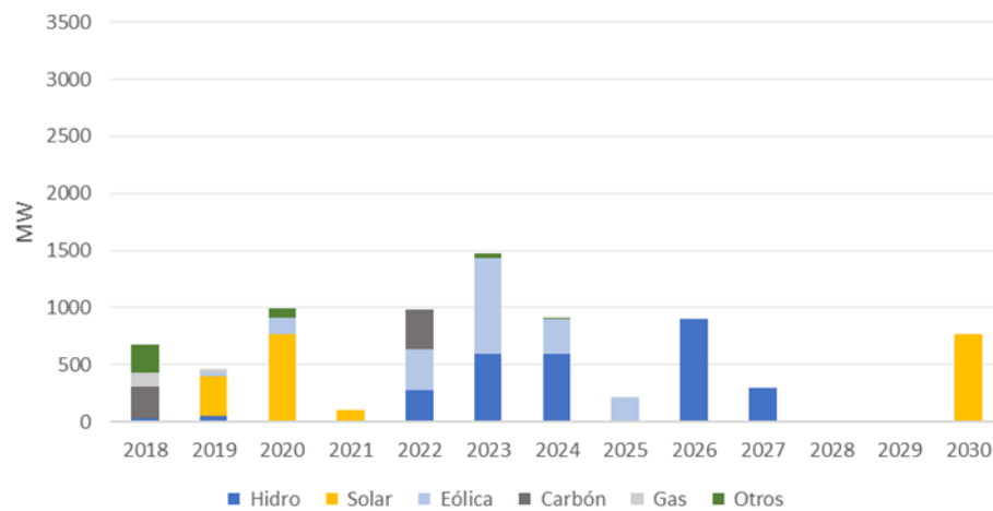
Figura 155 – Plan de Expansión sin la construcción de la línea HVDC Colectora 2 - Cerromatoso
