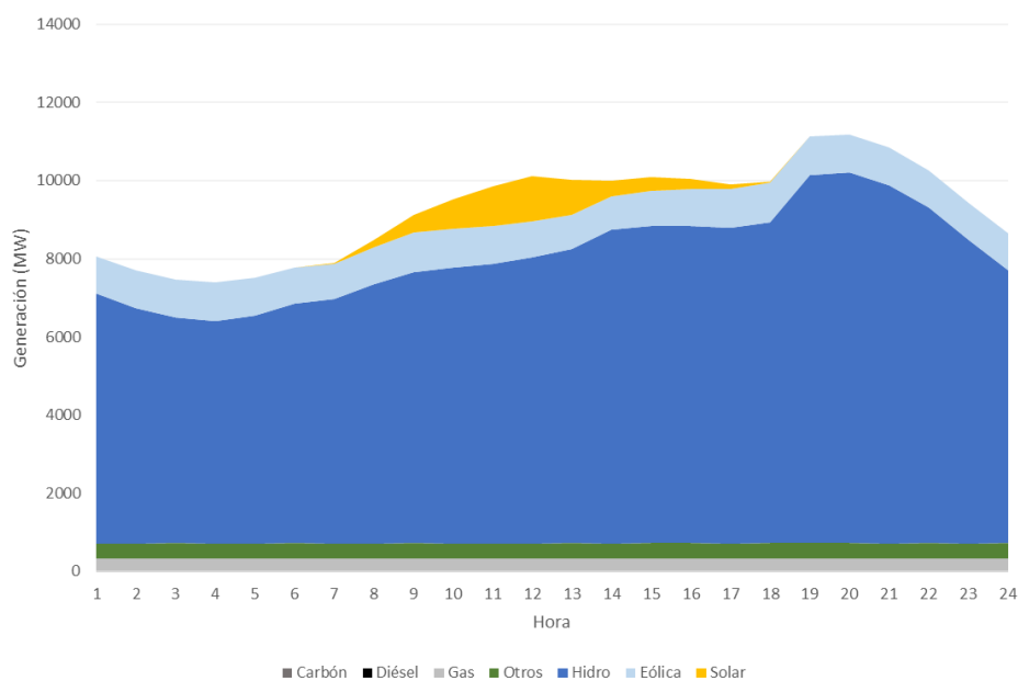
Figura 129 – Escenario con elevada GD, Balance Diario (Diciembre 2025, Hidrología Promedio).
