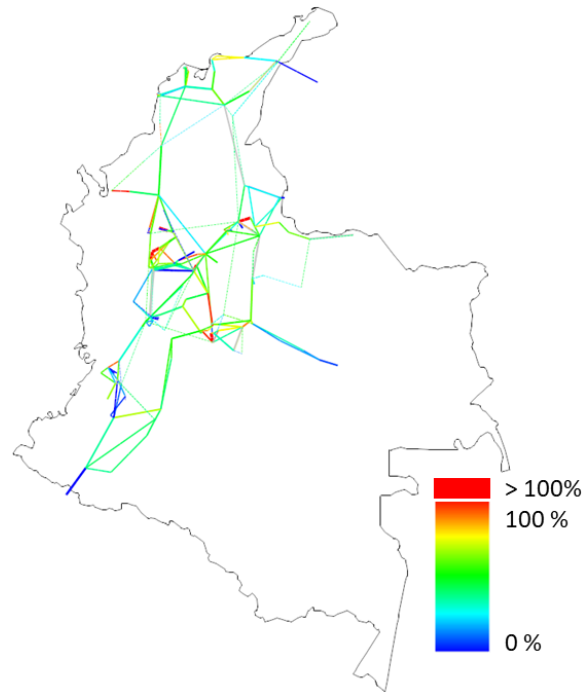
Figura 141 – flujo máximo en 2030 para el escenario de costo bajo de inversión para las renovables.
