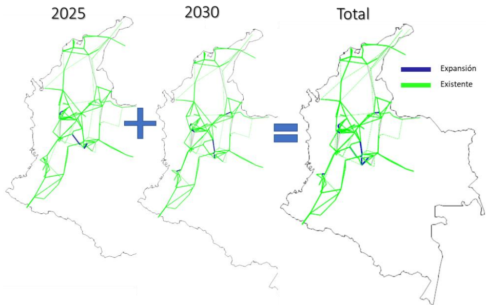
Figura 64 – Resultado de la expansión de transmisión para el escenario de referencia.
