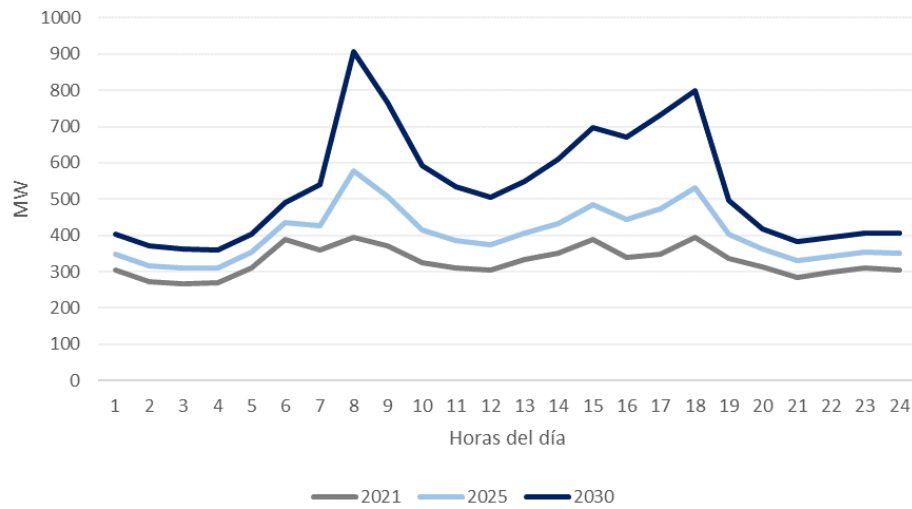
Figura 102 – Requerimientos de reserva en giro para la imprevisibilidad de las ERVs.
