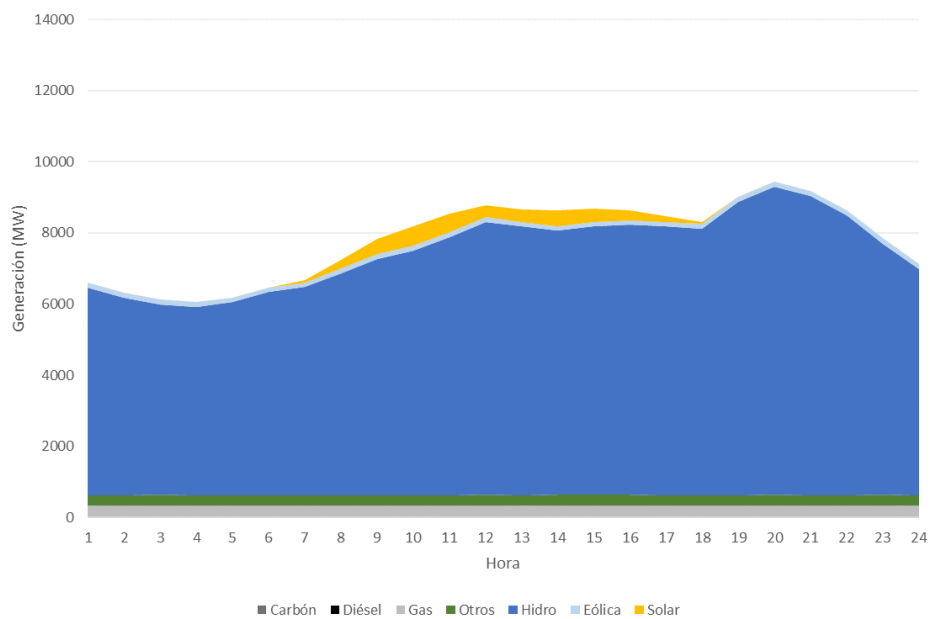
Figura 67 – Escenario de Referencia, Balance Diario (Junio 2021, Hidrología Promedio).
