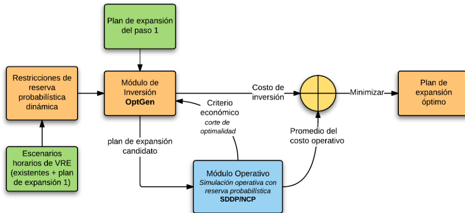
Figura 41 Planificación de las inversiones para el manejo de la variabilidad de las ERV
