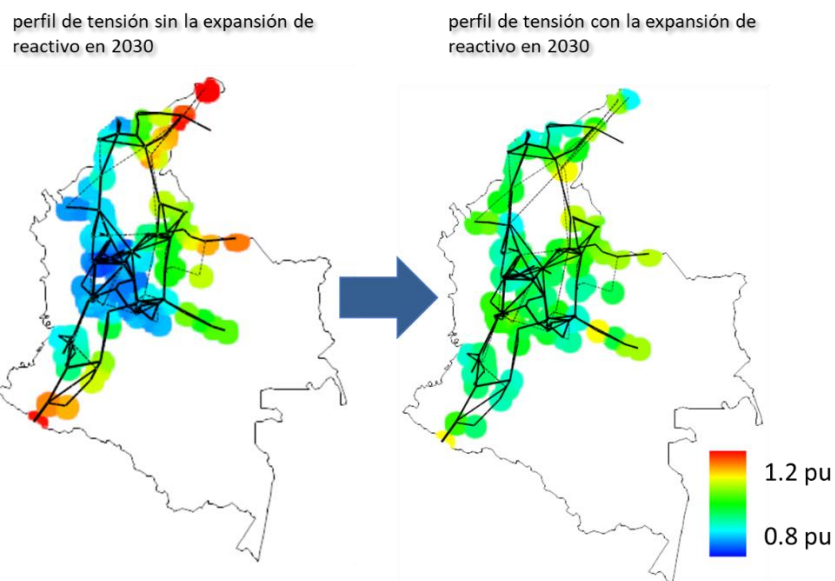
Figura 125 – Perfil de tensión sin la expansión x con la expansión en 2030 para el escenario de inserción agresiva de generación distribuida (Escenario Promedio, Diciembre).
