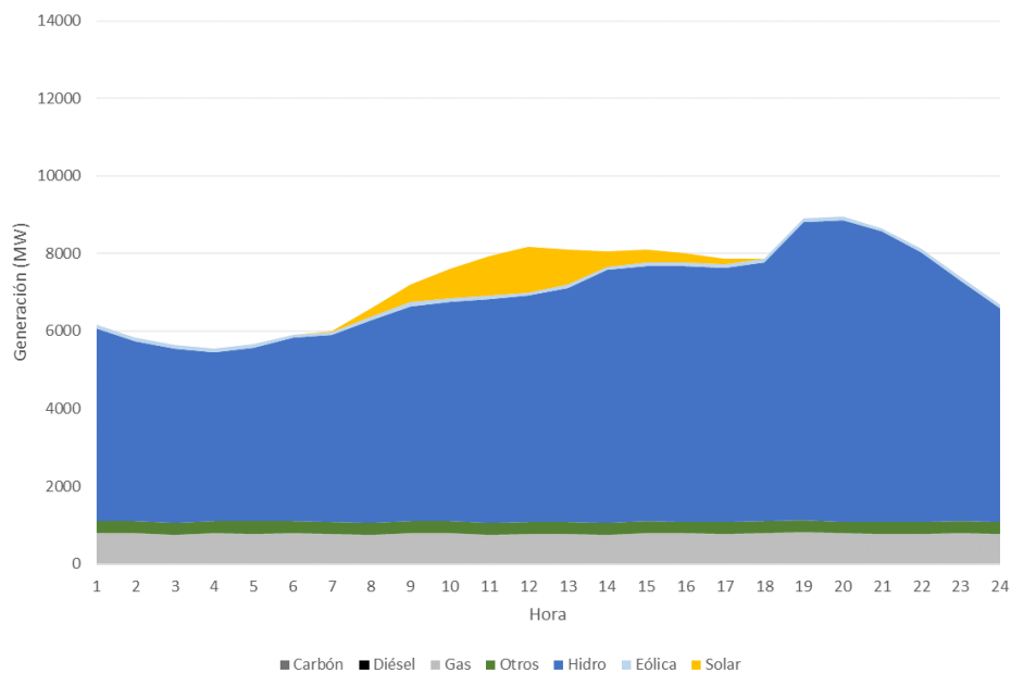
Figura 108 – Escenario sin Pescadero, Balance Diario (Diciembre 2021, Hidrología Promedio).
