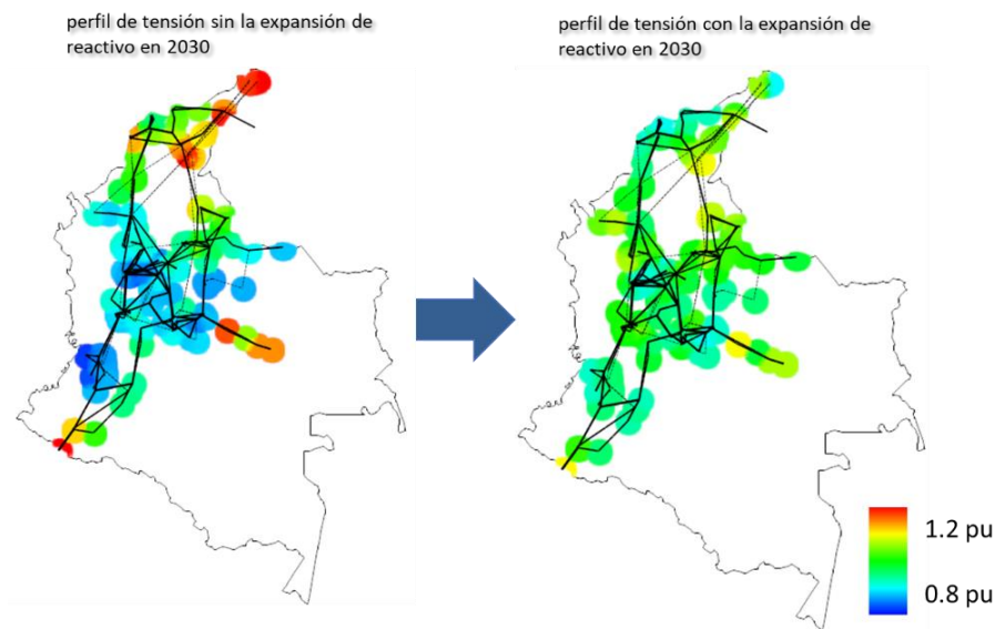
Figura 87 – Perfil de tensión sin la expansión x con la expansión en 2030 para el escenario de demanda alta (Escenario Promedio, Diciembre).
