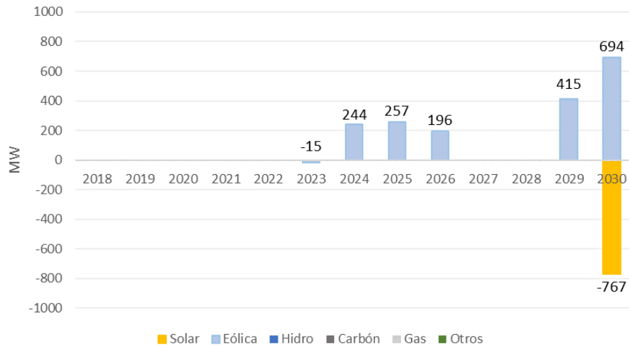
Figura 156 – Comparación año x año de los planes de expansión, con y sin la interconexión HVDC Colectora 2 - Cerromatoso
