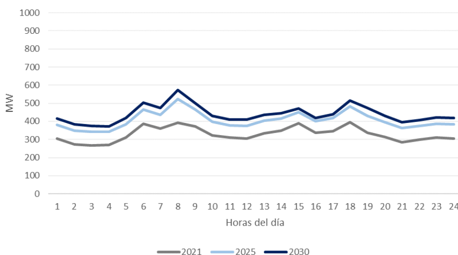
Figura 83 –Requerimientos de reserva para la imprevisibilidad de las ERVs.
