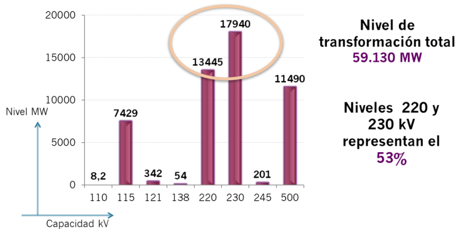
Figura 4 – Capacidad de transformación por nivel de voltaje
