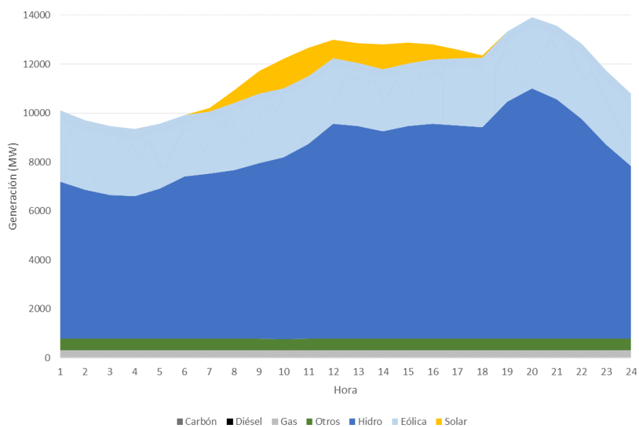
Figura 149 – Escenario precios bajos renovables, Balance Diario (Junio 2030, Hidrología Promedio).
