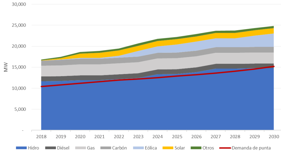
Figura 118 – Balance de Potencia por año – Escenario con elevada GD
