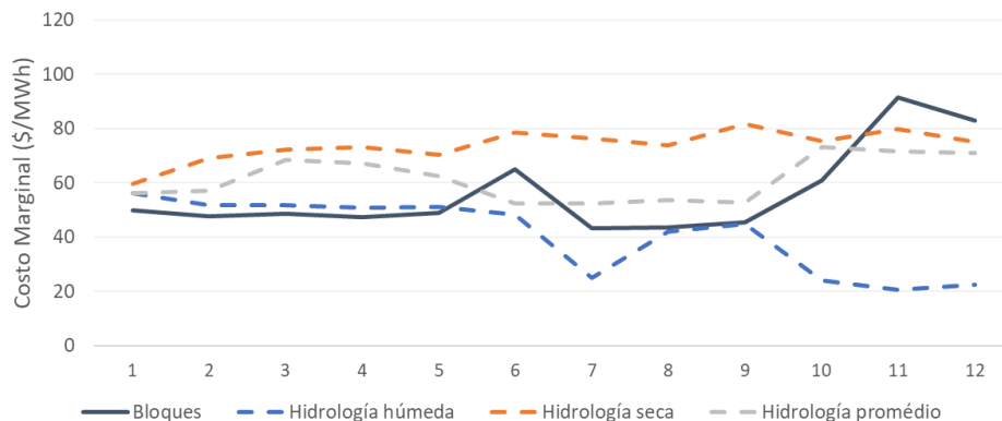
Figura 73 – Escenario de Referencia, Costos marginales horarios (2021).
