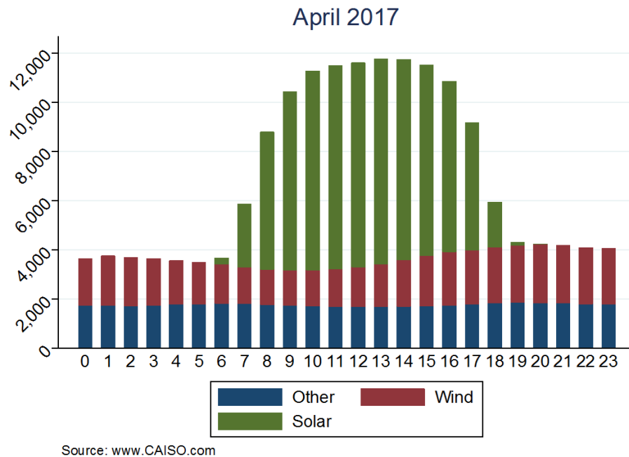
Figura 28 – Perfil diario típico de producción (California) - 2017
