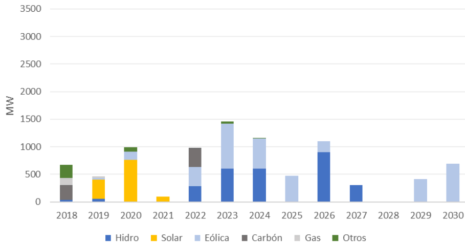
Figura 154 – Plan de Expansión con la construcción de la línea HVDC Colectora 2 – Cerromatoso (2023)
