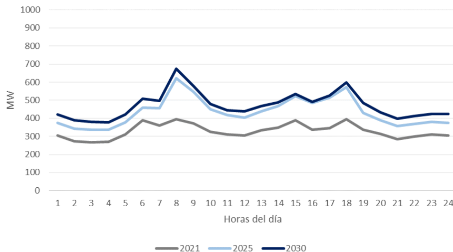
Figura 140 – requerimientos de reserva en giro para la imprevisibilidad de las ERVs.
