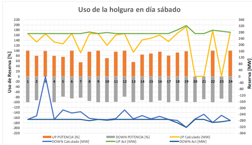
Figura 17 – Holgura AGC en días sábado
