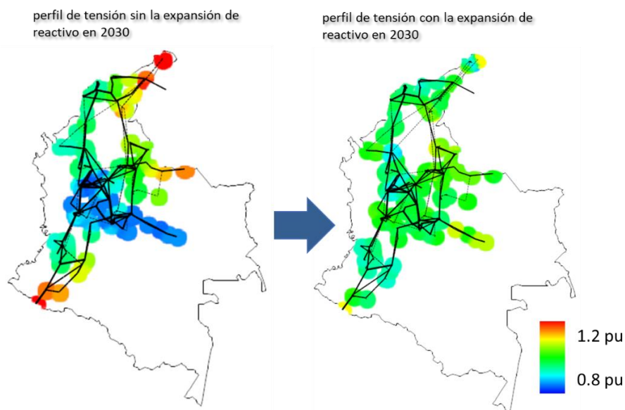
Figura 106 – Perfil de tensión sin la expansión x con la expansión en 2030 para el escenario sin Pescadero/Ituango (Escenario Promedio, Diciembre).
