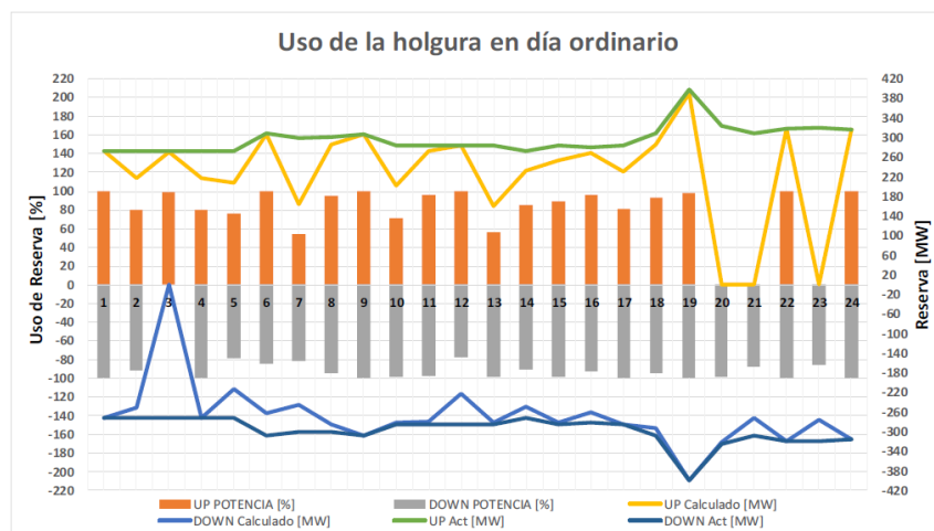
Figura 165 – Holgura AGC en días ordinarios
