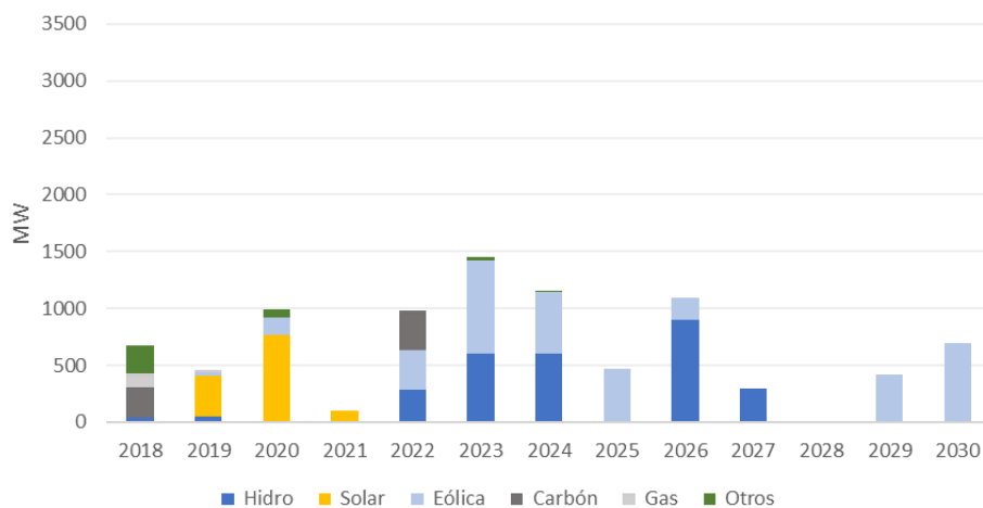
Figura 57 – Adición de capacidad por año – Escenario de Referencia.
