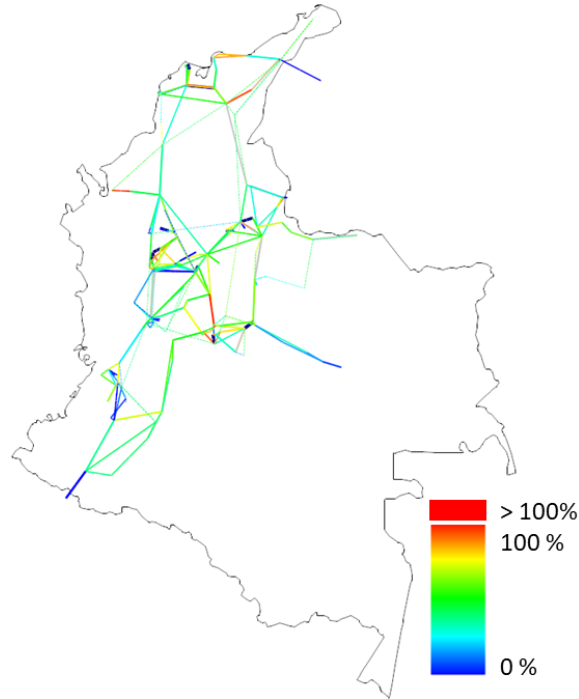
Figura 103 – flujo máximo en 2030 para el escenario sin Pescadero/Ituango.
