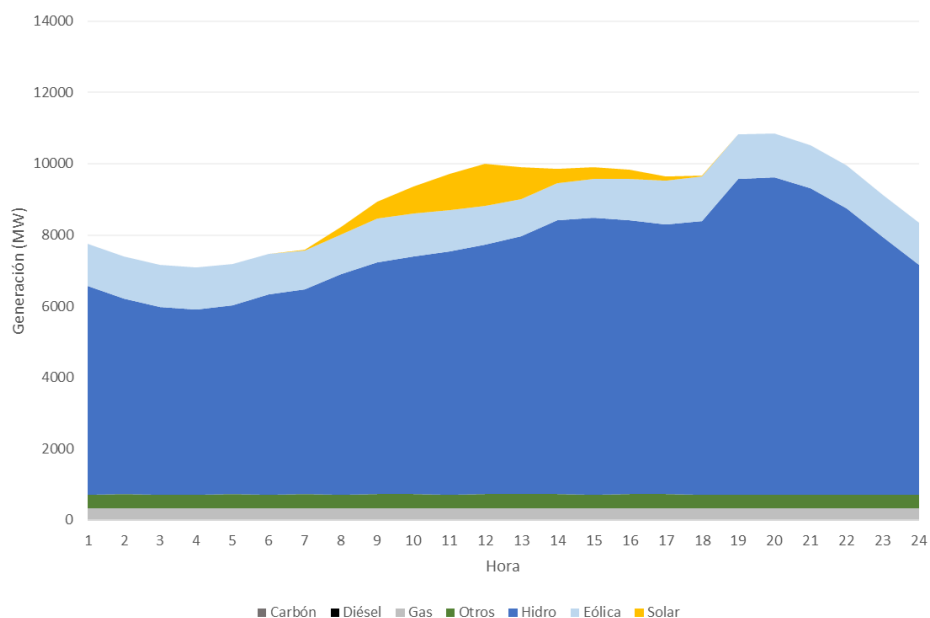
Figura 70 – Escenario de Referencia, Balance Diario (Diciembre 2025, Hidrología Promedio).
