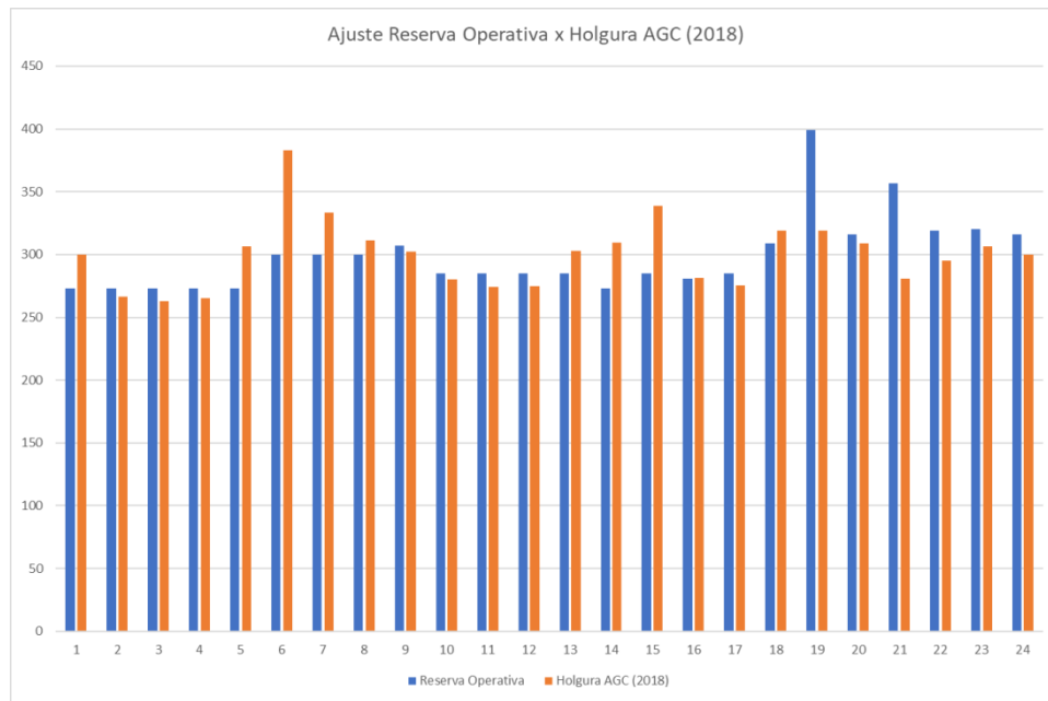
Figura 172 – Ajuste reserva operativa en función de la holgura AGC para 2018
