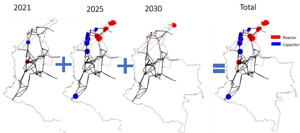
Figura 124 – Resultado de la expansión de reactivo para el escenario inserción agresiva de generación distribuida.
