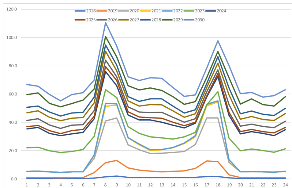
Figura 170 – Reserva para el manejo de las renovables (asume la inserción del escenario base)
