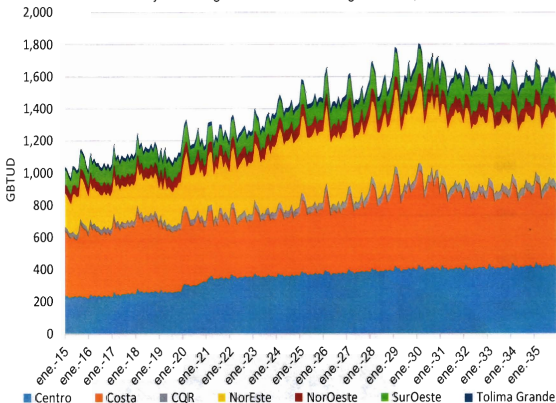
Gráfica 2-17 Proyección regional de demanda de gas natural, escenario medio.
