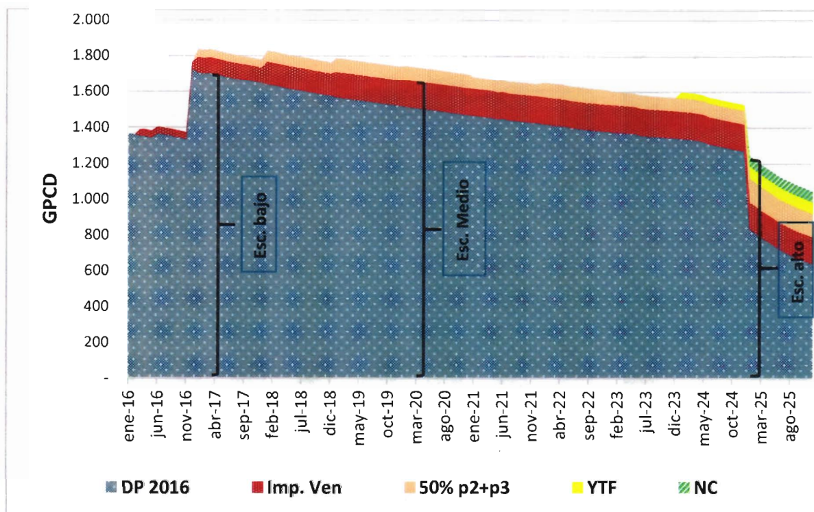
Gráfica 1-9. Escenarios de oferta de gas natural
