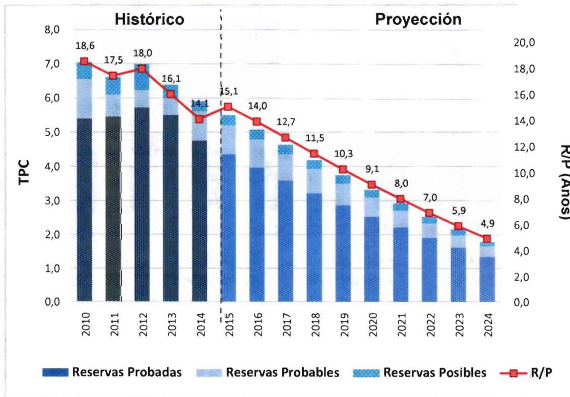
Gráfica 1-2. Comportamiento reservas gas natural
