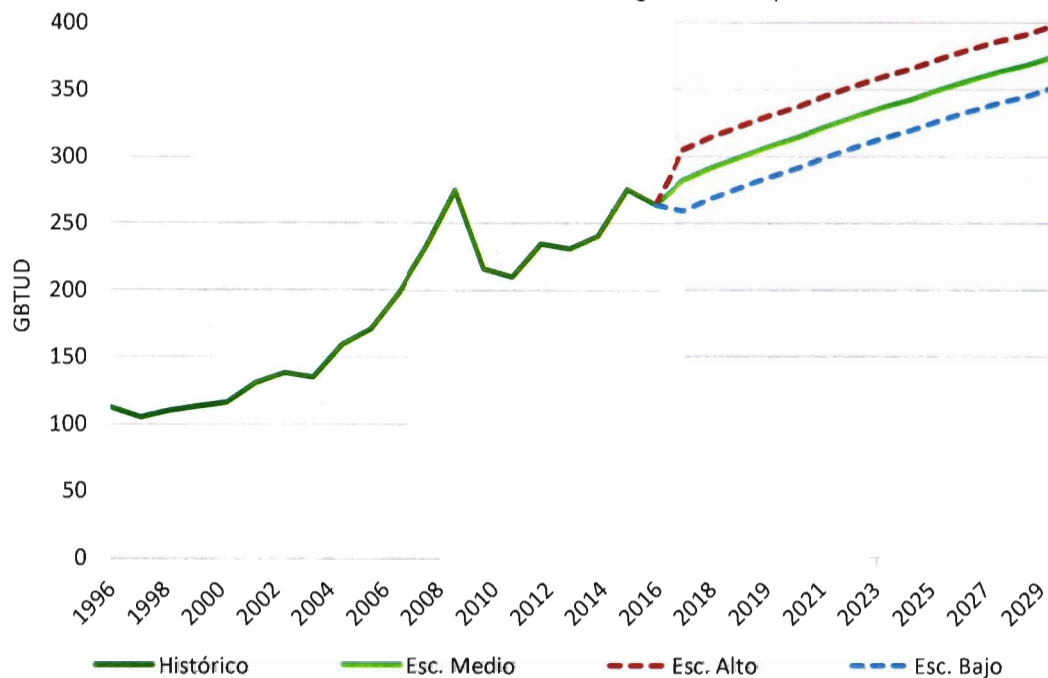
Gráfica 2-8: Escenarios de demanda nacional de gas natural para el sector industrial
