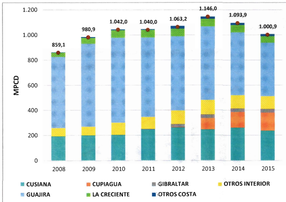
Gráfica 1-3. Producción de gas natural
