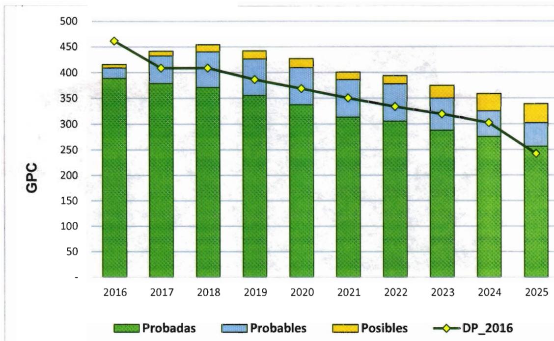
Gráfica 1-8. Producción de reservas Vs declaración de producción 2016
