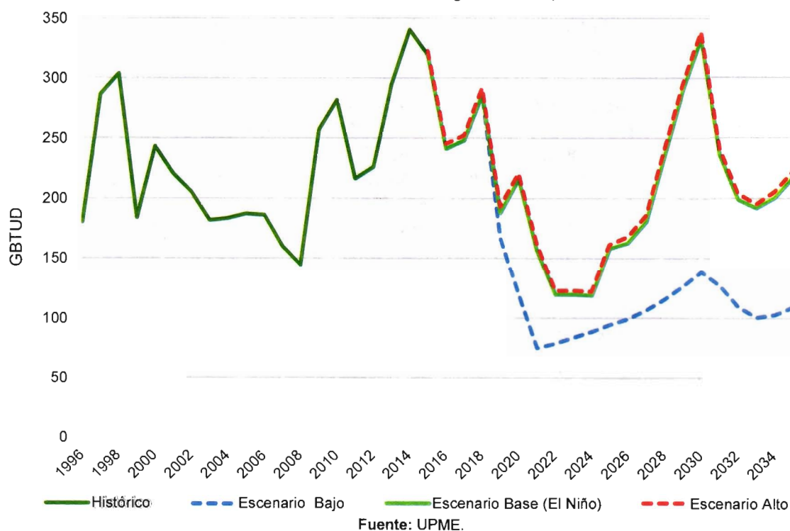
Gráfica 2-14 Escenarios de demanda nacional de gas natural para el sector termoeléctrico.
