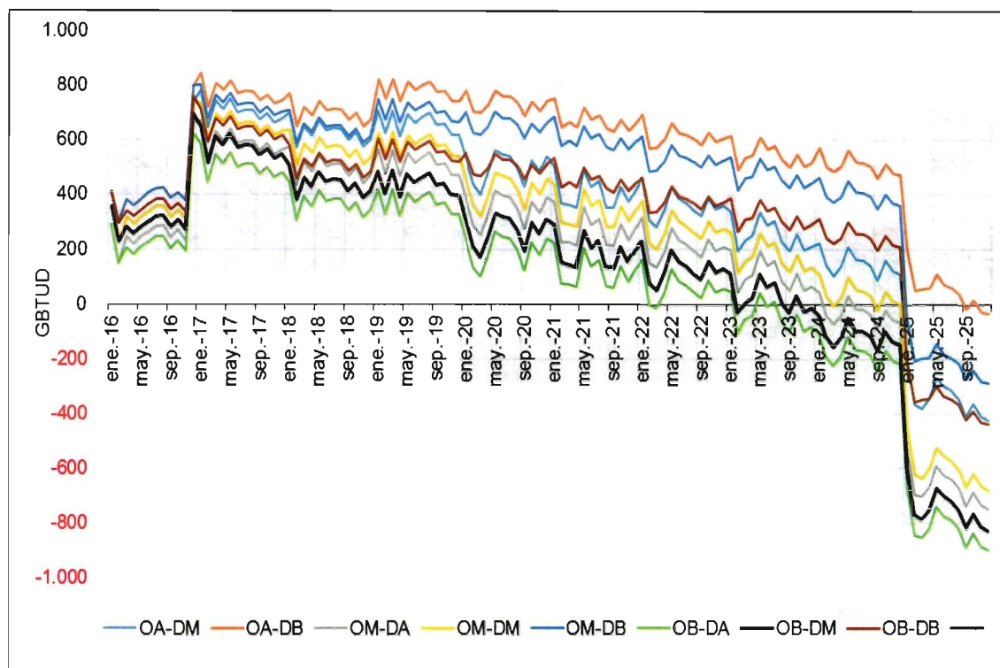
Gráfica 3-2. Balance de gas natural (Superávit y Déficit)
