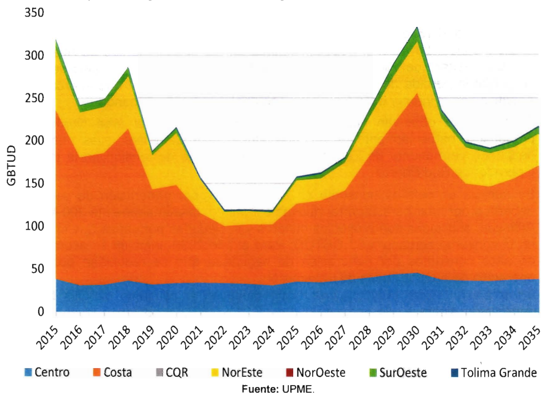
Gráfica 2-14 Escenarios de demanda nacional de gas natural para el sector termoeléctrico.
