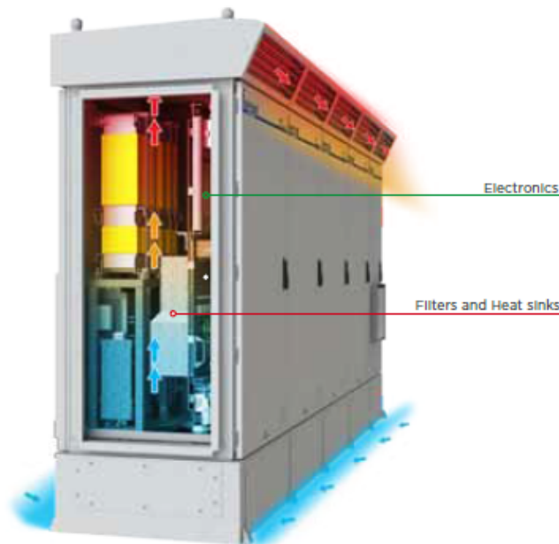
Figura 19. Imagen de inversor centralizado intemperie facilitada por Power-Electronics
