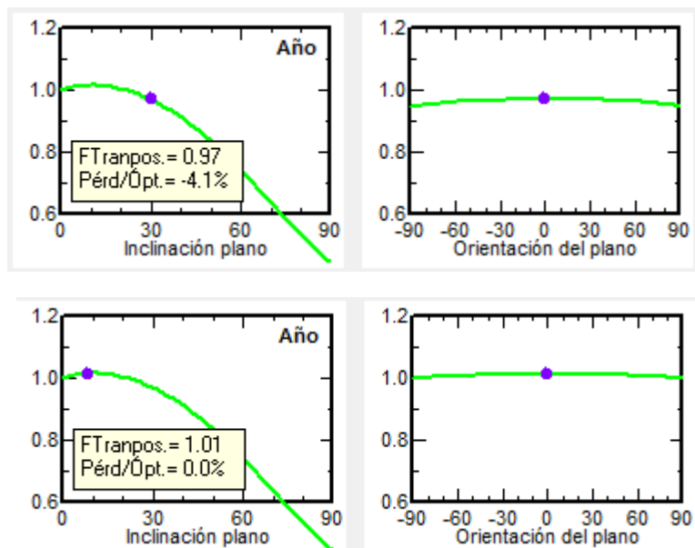
Figura 9. Imágenes correspondientes al software PVSYST de una simulación en Colombia
